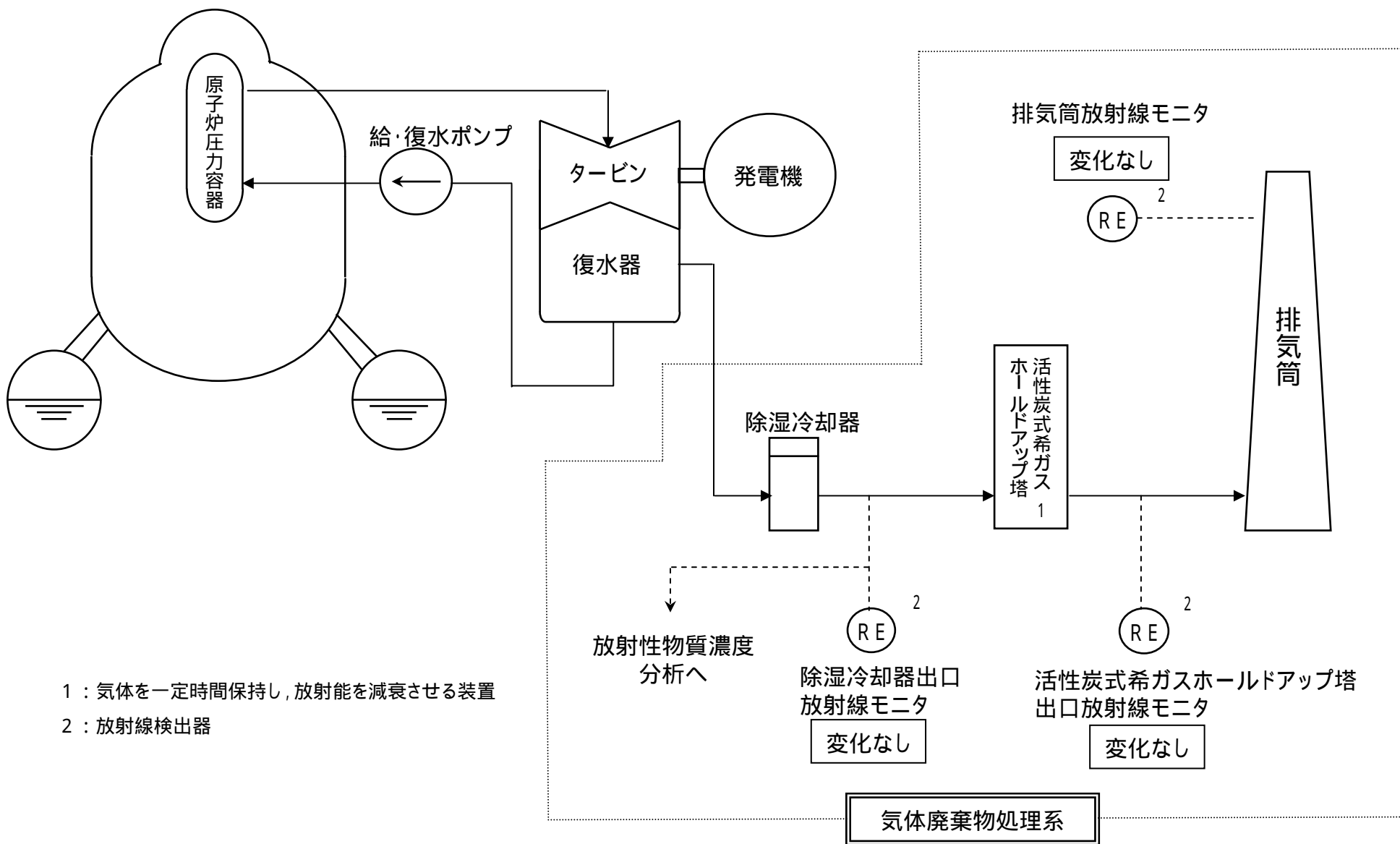
女川3号機気体廃棄物処理系系統概略図
