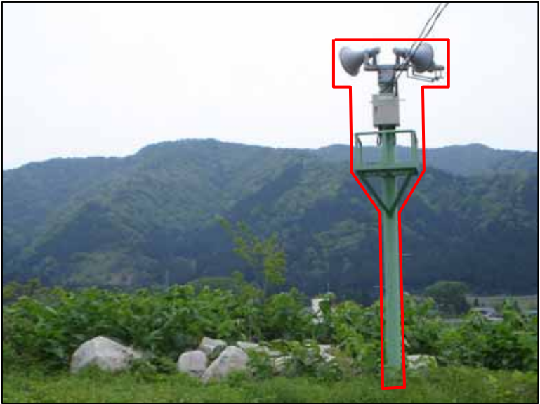
写真4 放流警報装置の設置 (阿賀野川水系阿賀野川:新潟県五泉市) 関係発電所:揚川発電所
