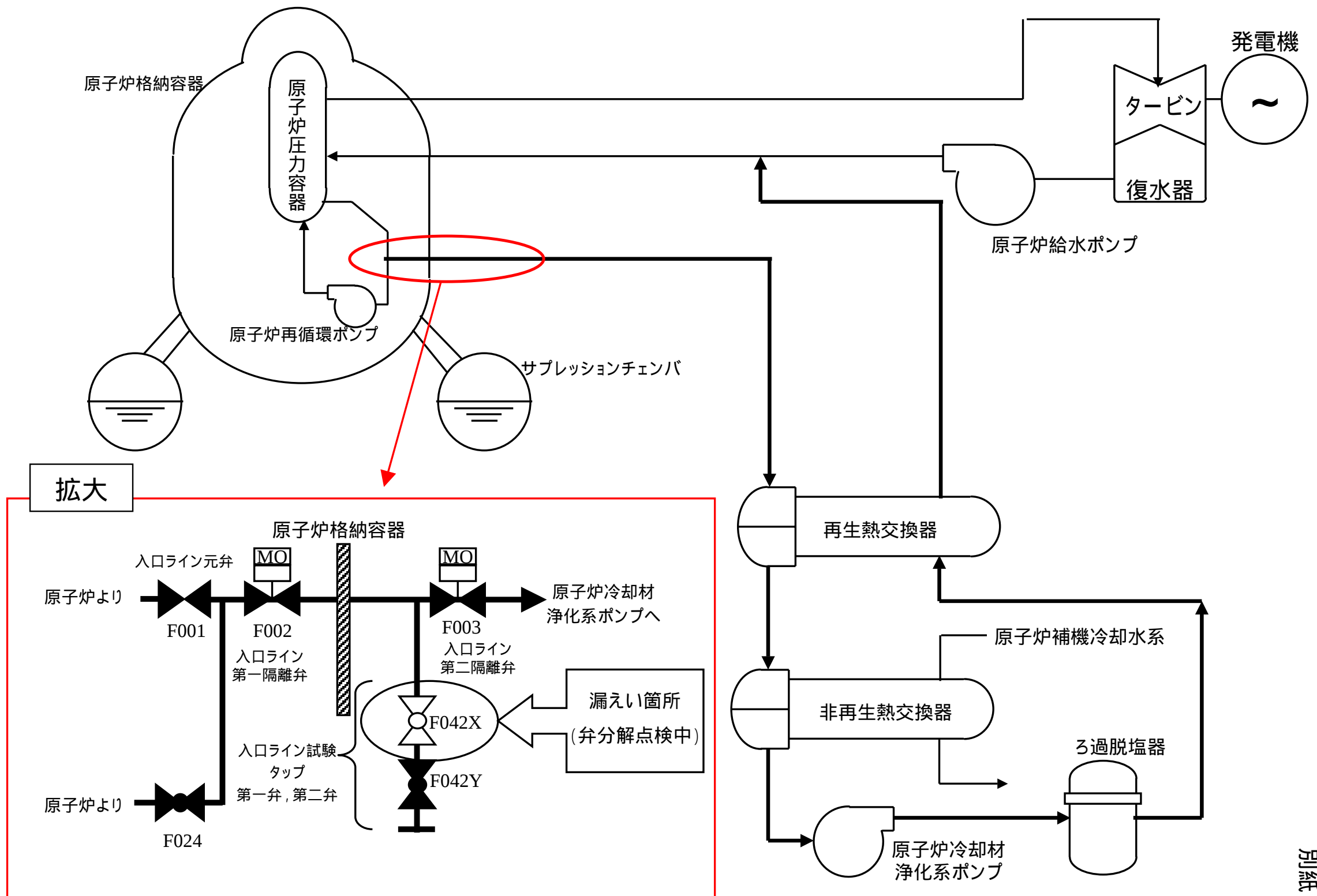
女川2号機 原子炉冷却材浄化系 系統概要図
