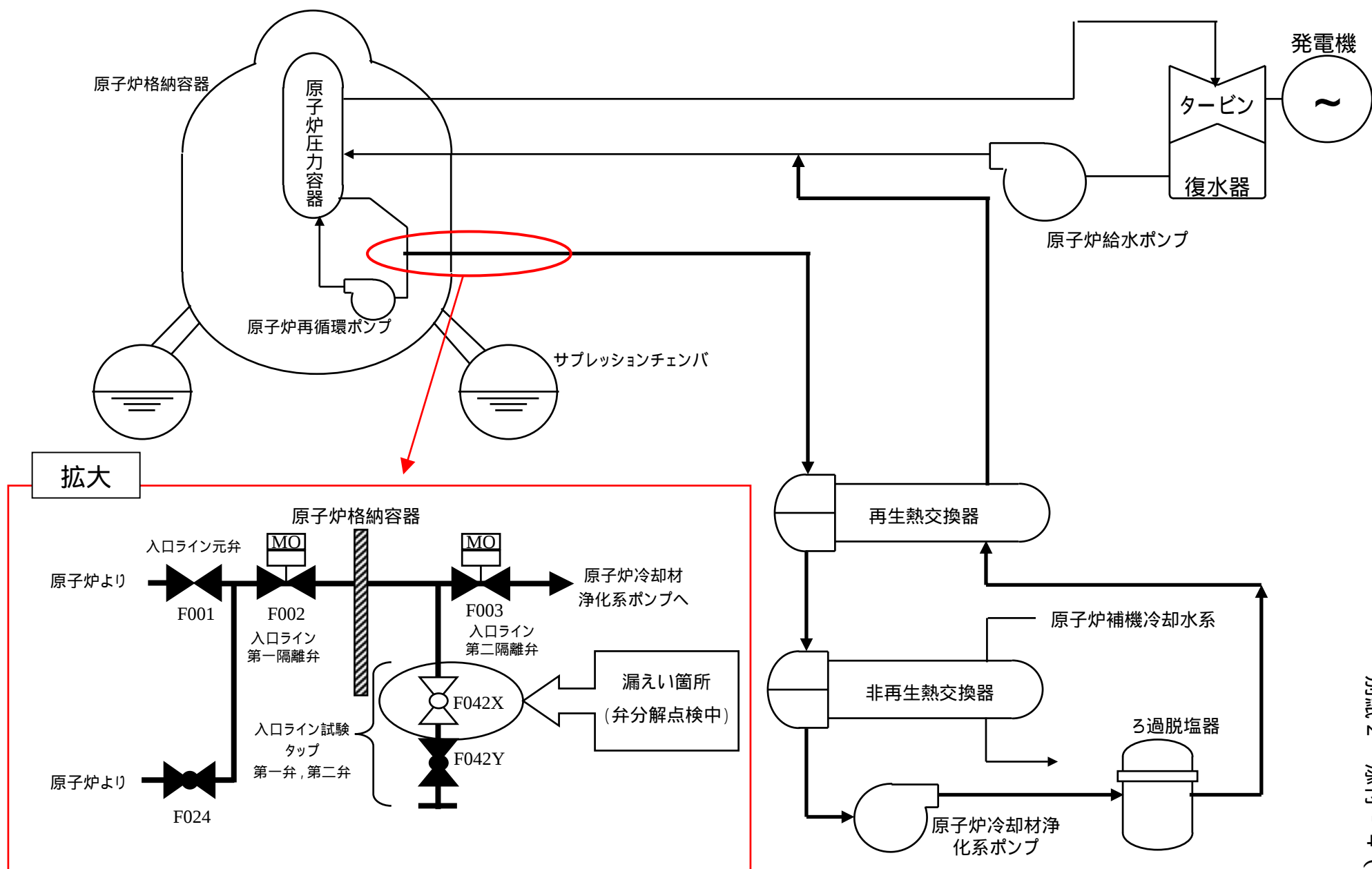
女川2号機 原子炉冷却材浄化系 系統概要図
