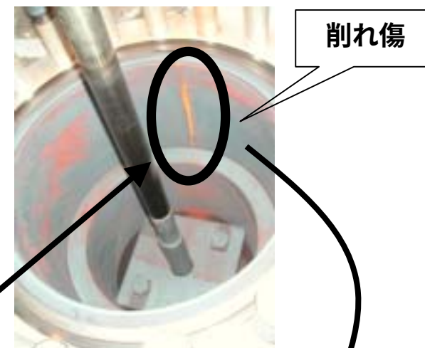
弁箱（下側）
