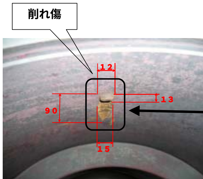
弁箱（上側）
