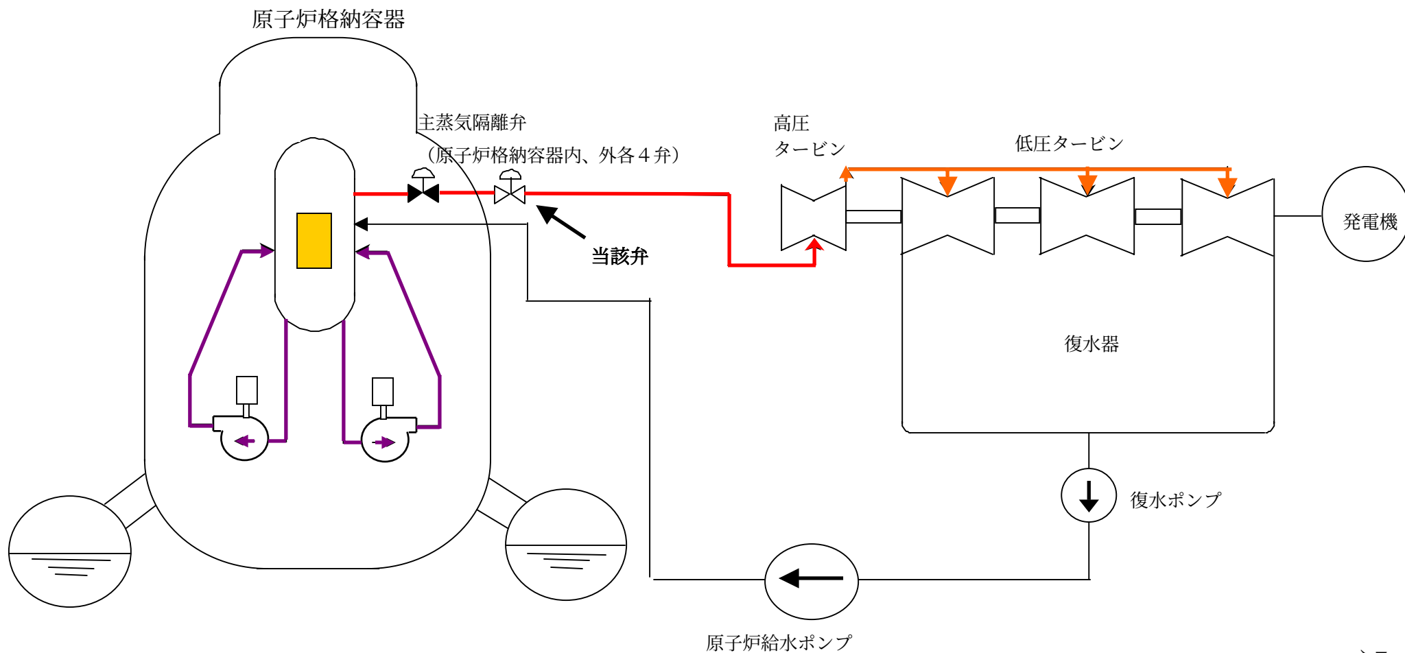
系統概略図
