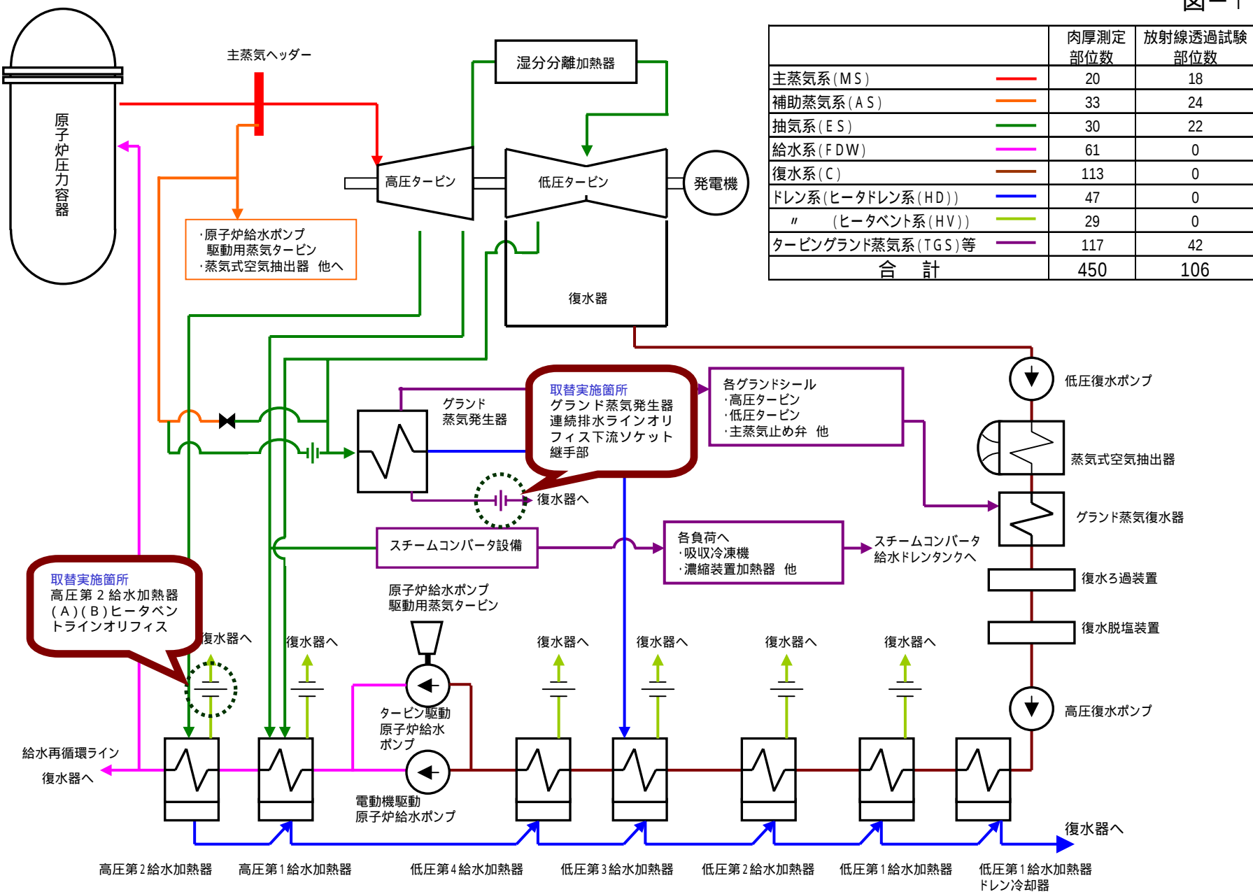
女川原子力発電所2号機系統概略図
