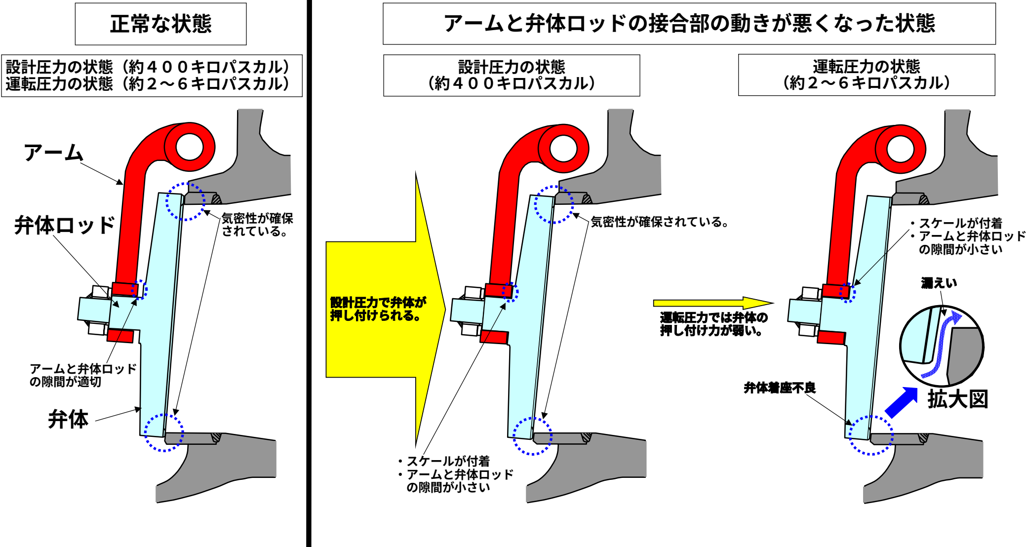
高圧注水系タービン排気ライン逆止弁 概略図
