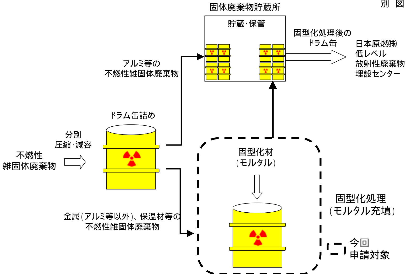
不燃性雑固体廃棄物の固型化処理の概要
