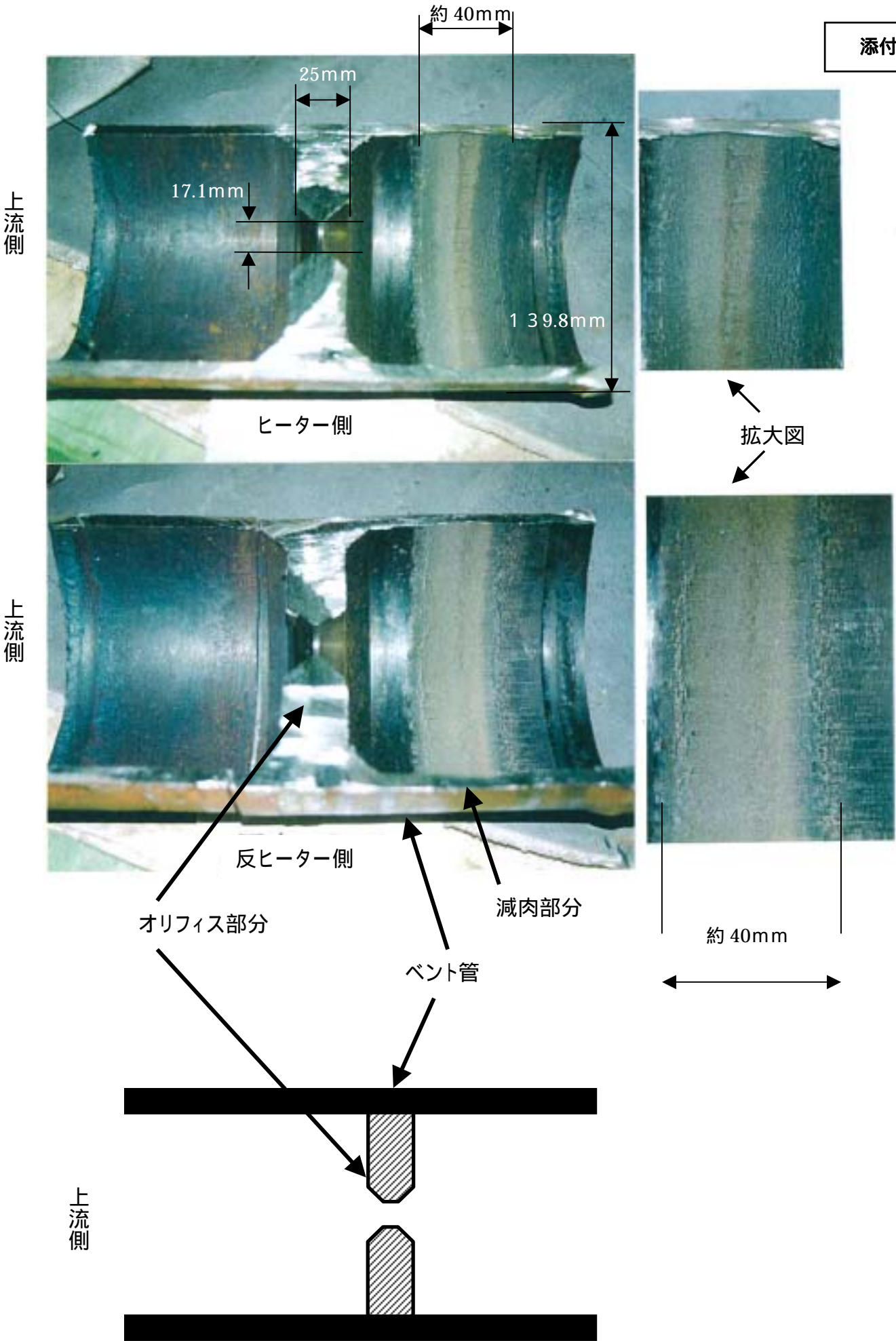
減肉の状況 【例：2号機高圧第1給水加熱器(A)】
