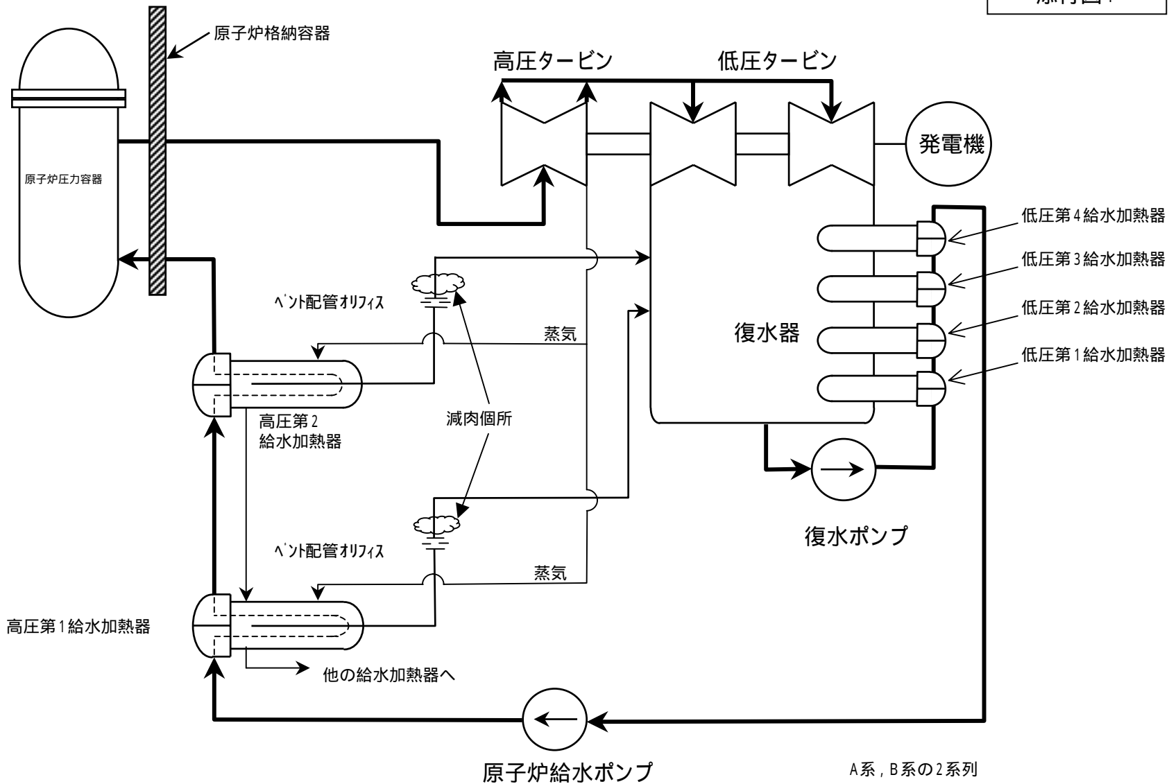
高圧給水加熱器概略系統図
