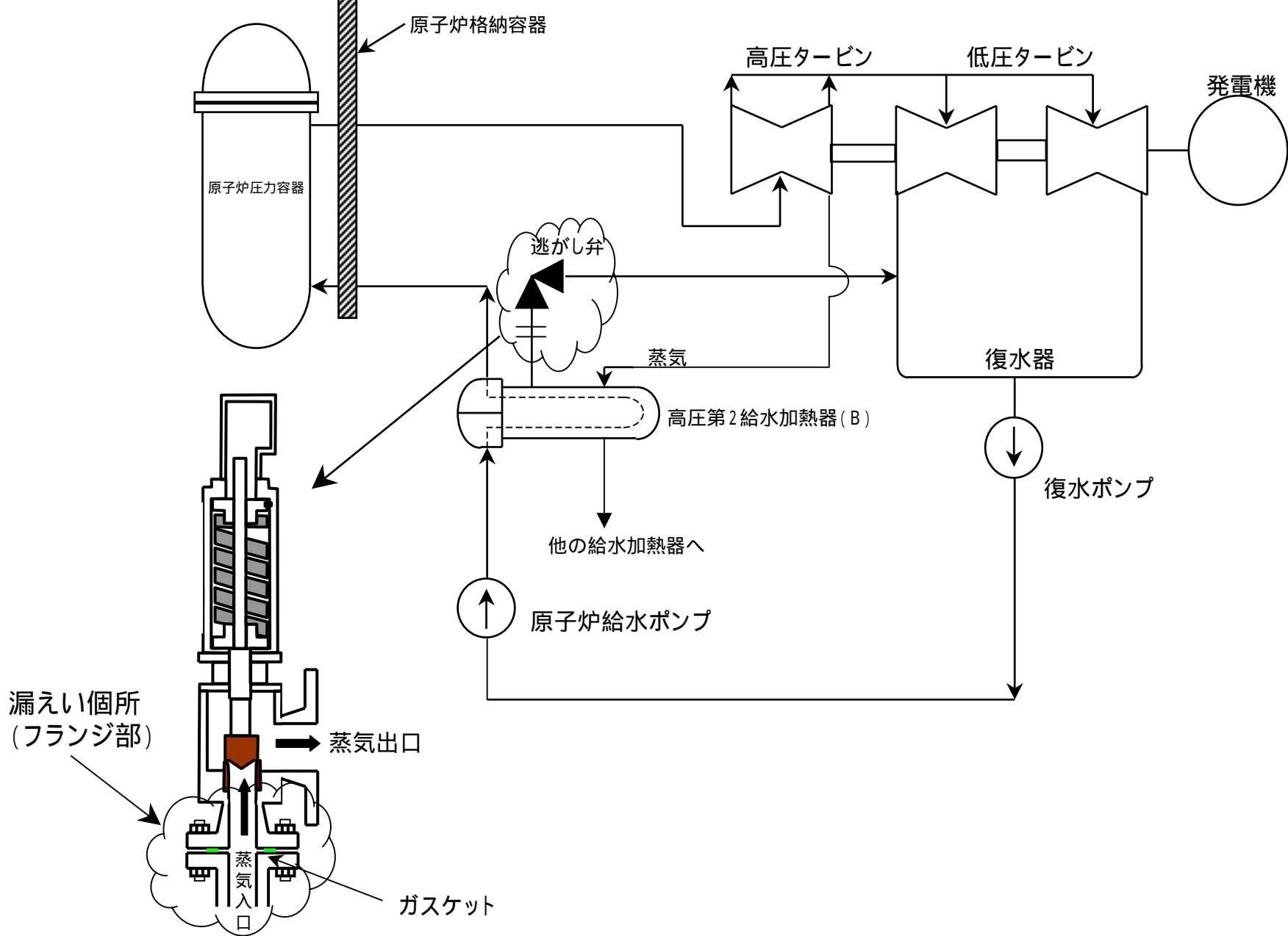
高圧第2給水加熱器(B)概略系統図および逃がし弁概略図
