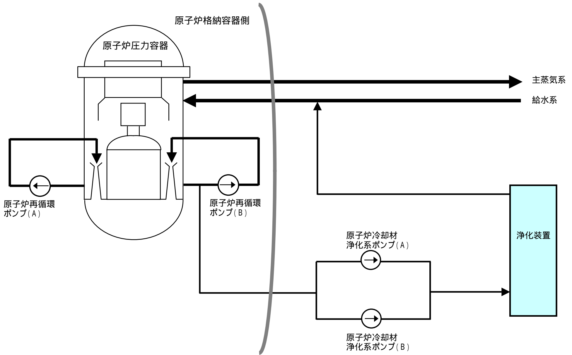
原子炉冷却材浄化系系統概略図
