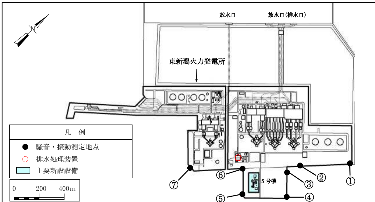
騒音・振動測定位置図
