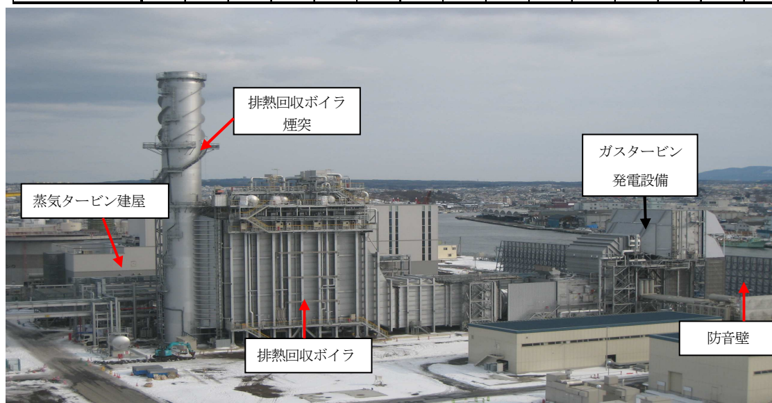
排熱回収ボイラ据付・蒸気タービン建屋工事（平成 26 年 2 月 14 日撮影）
