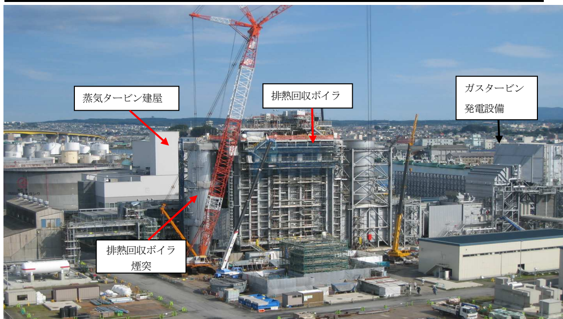
排熱回収ボイラ据付・蒸気タービン建屋工事（平成 25 年 9 月 9 日撮影）
