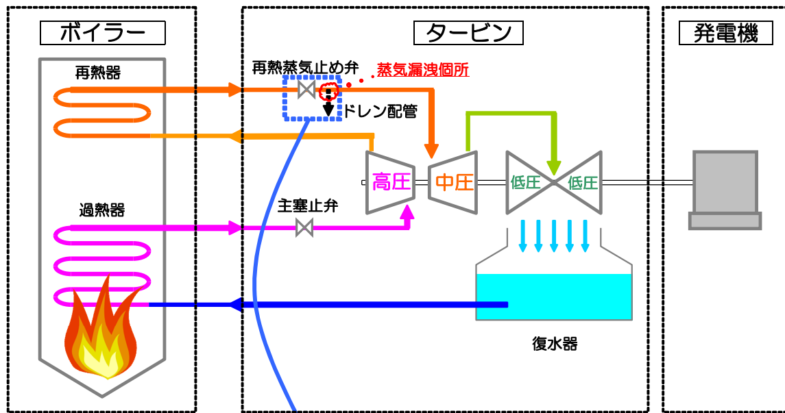
蒸気配管系統概略図
