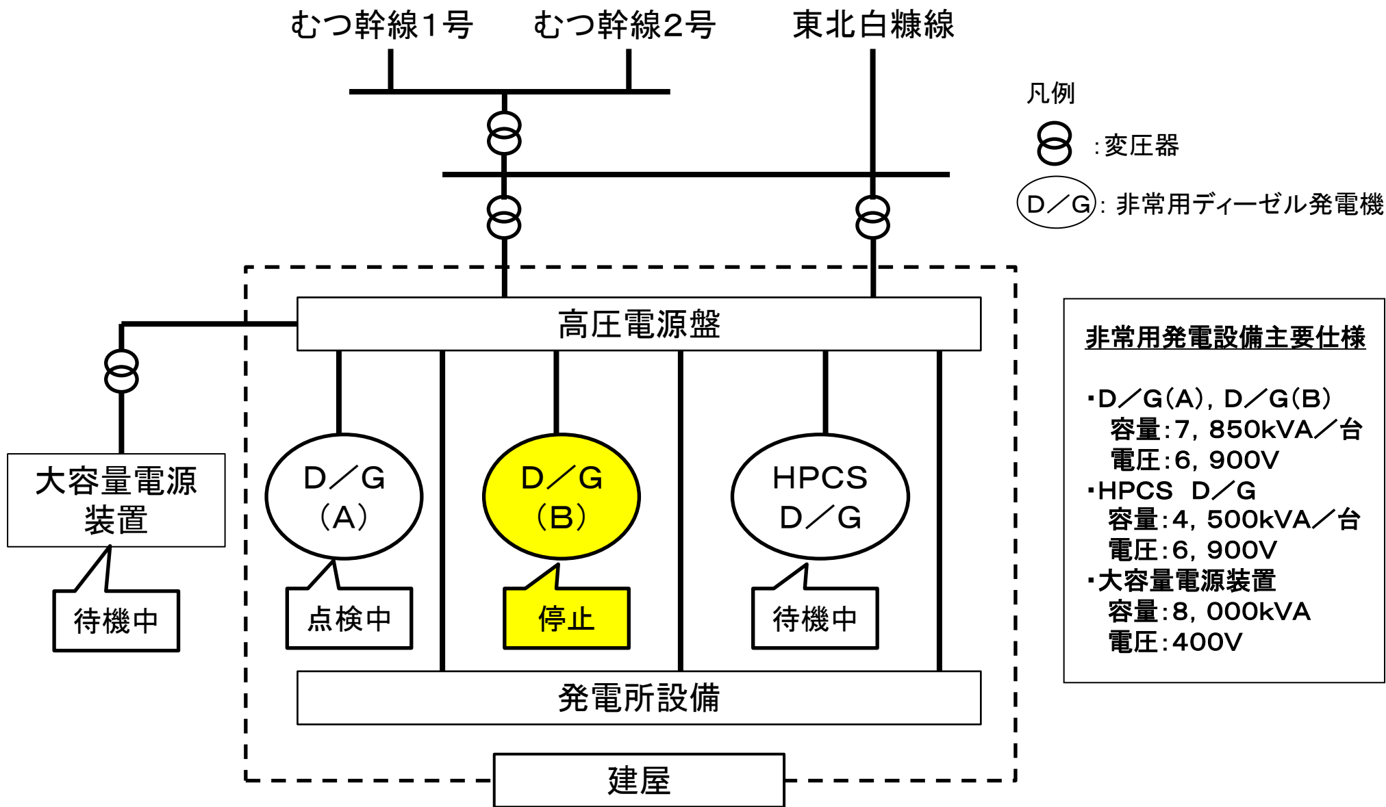
東通原子力発電所1号機の電源系統の状態
