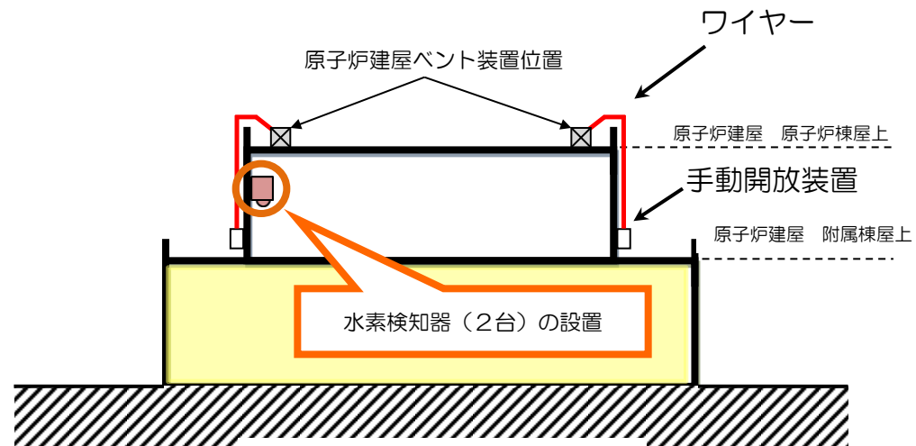
&lt;原子炉建屋 断面図&gt;
