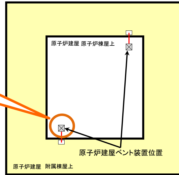
&lt;原子炉建屋 屋上平面図&gt;
