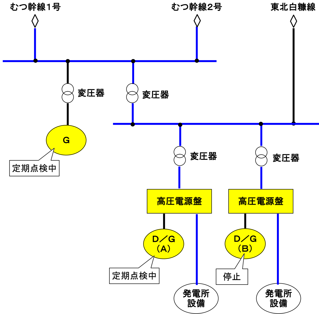
東通原子力発電所1号機の電源系統状態
