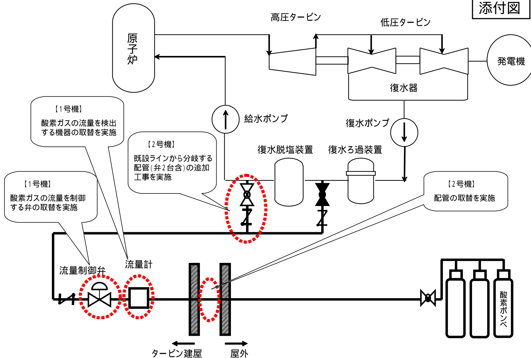
酸素注入系概略系統図
