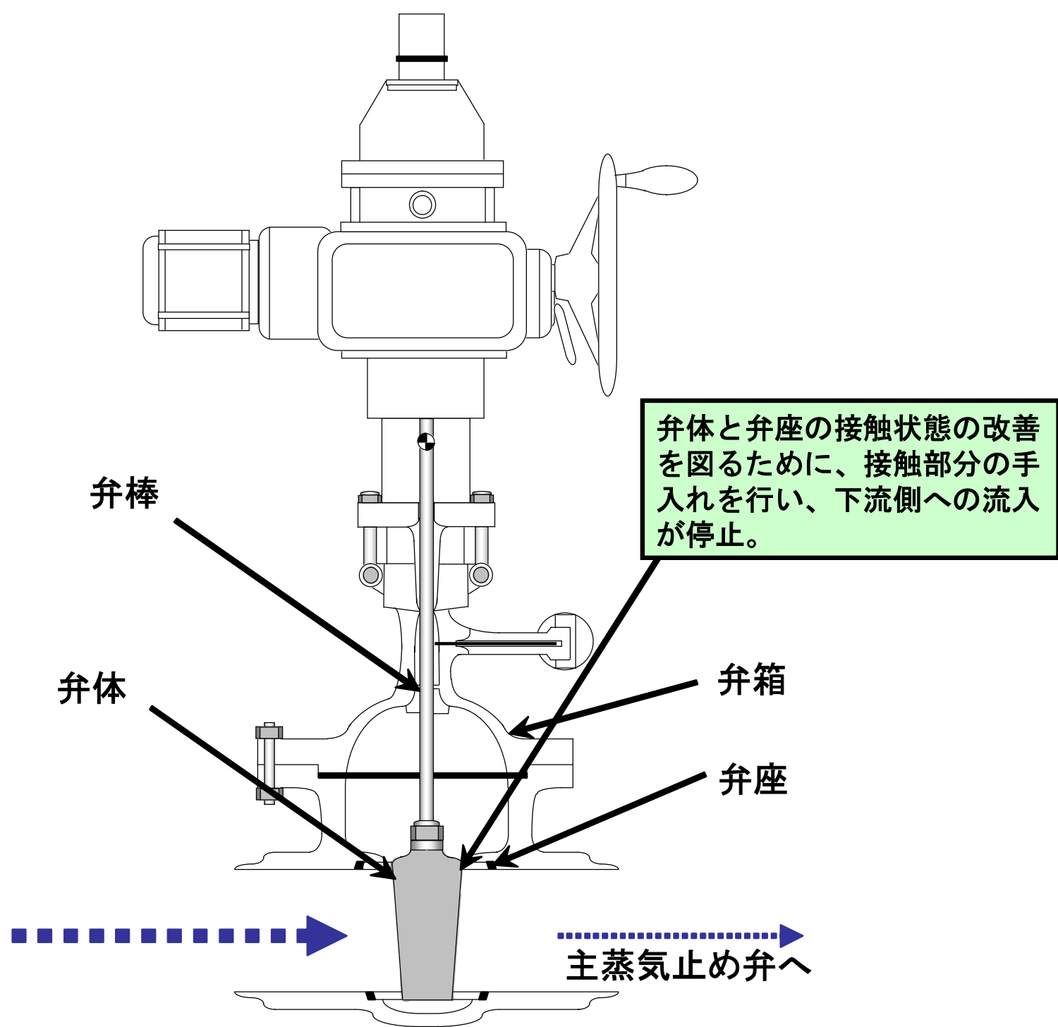
高圧注水系ポンプ駆動用タービン止め弁概念図
