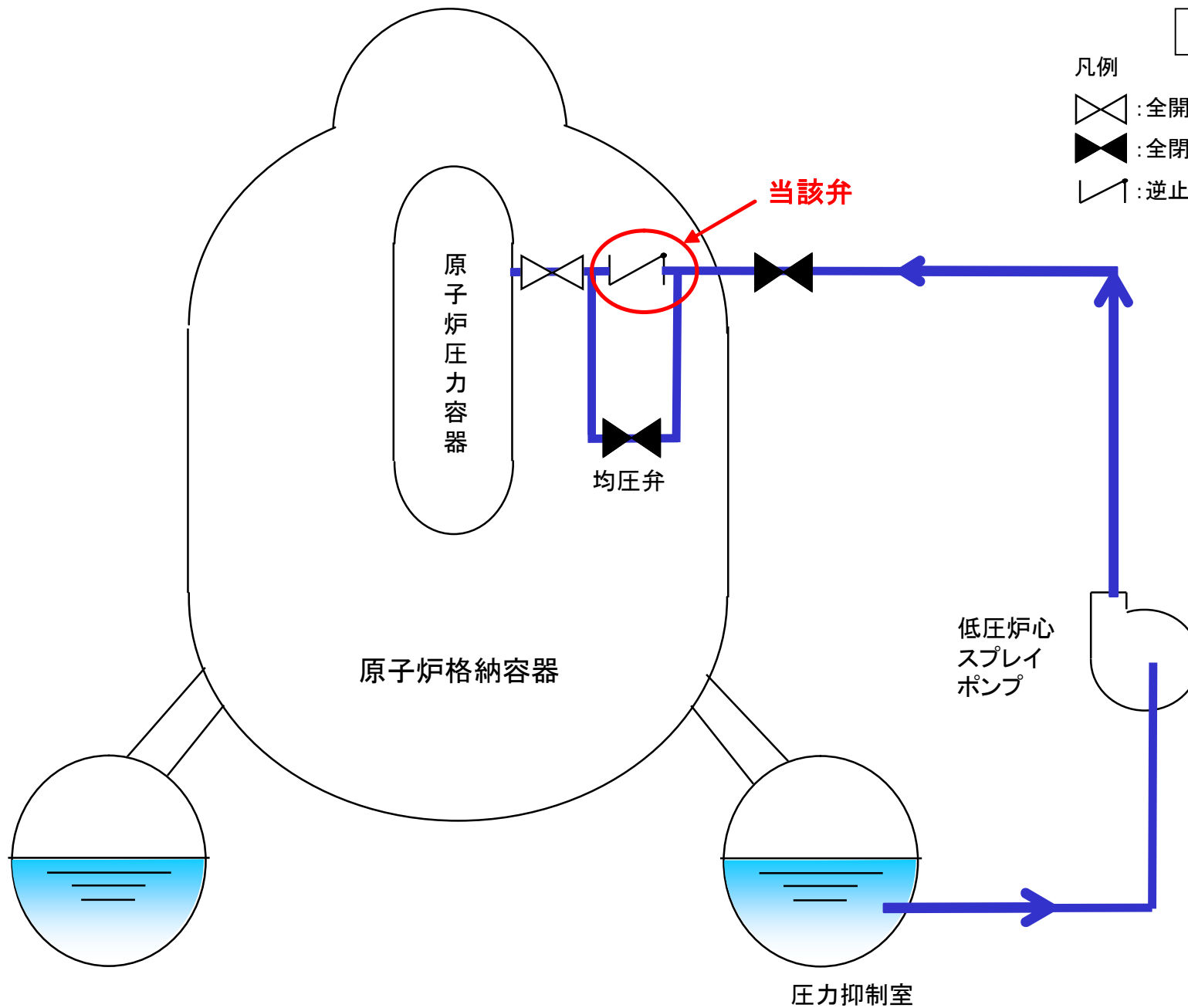
低圧炉心スプレイ系 系統概要図
