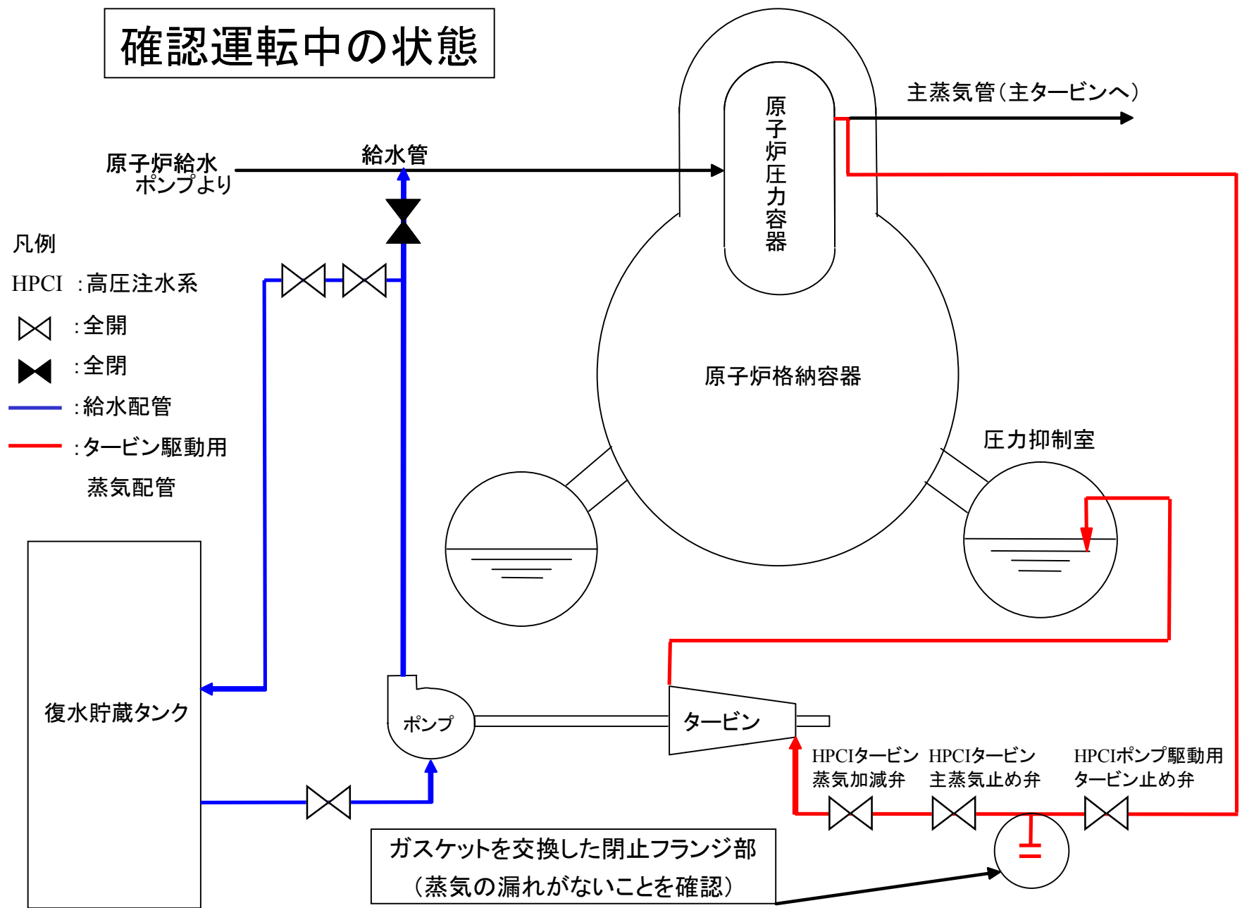
高圧注水系 系統概要図
