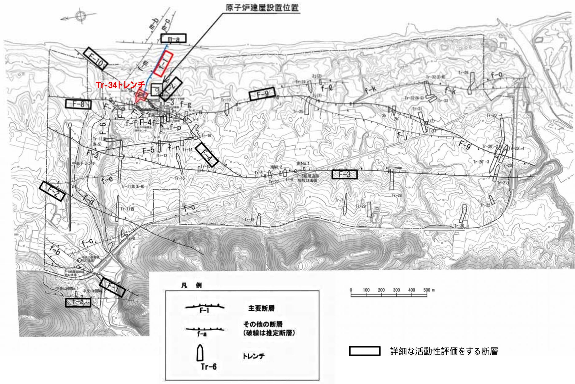
東通原子力発電所の敷地内断層の位置図 (f - 1断層と調査用のTr - 34トレンチの位置)
