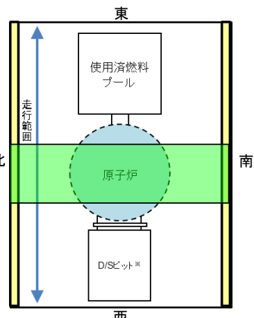
原子炉建屋5階平面図
