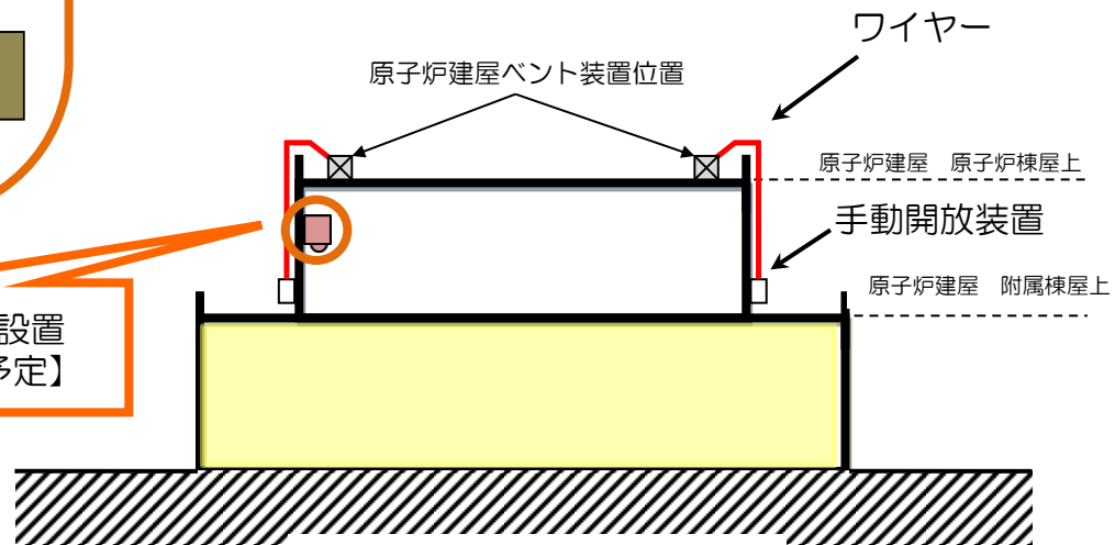
<原子炉建屋 断面図>
