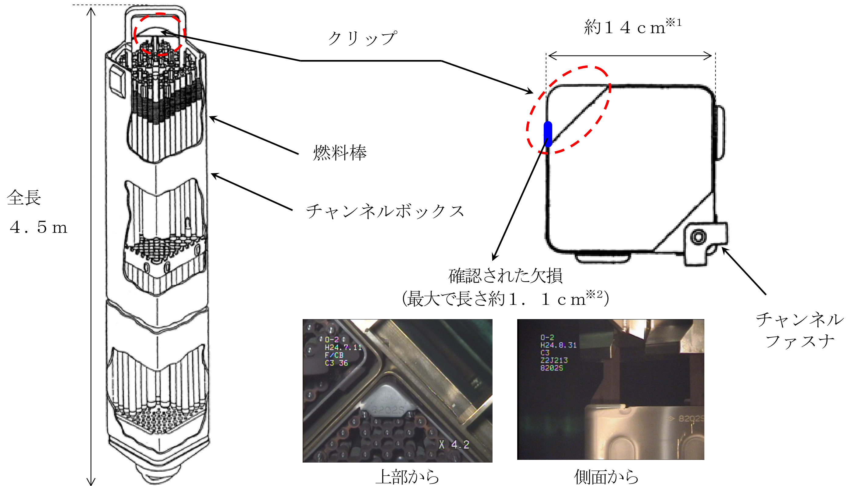
燃料集合体概要図
