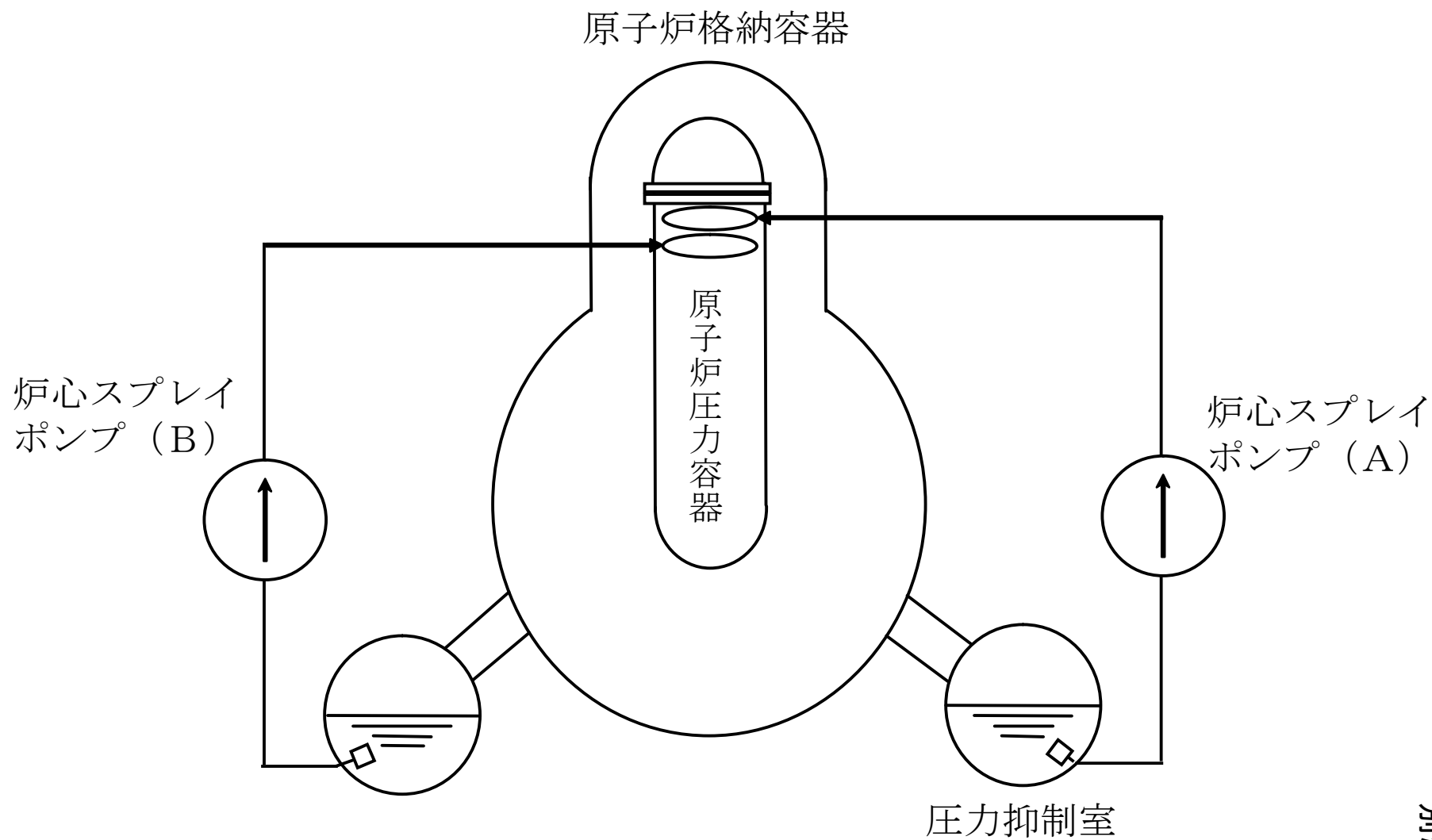
炉心スプレイ系 系統概要図
