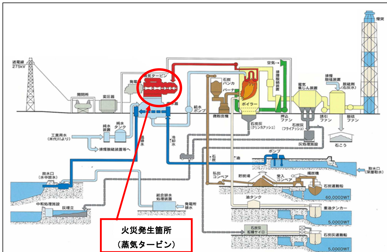
■能代火力発電所 1 号機 概略図
