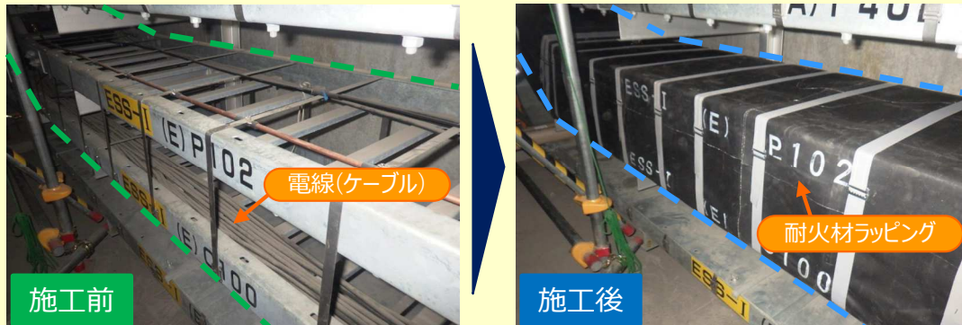
【順次実施している「ケーブルトレイへの耐火材ラッピング工事」】
