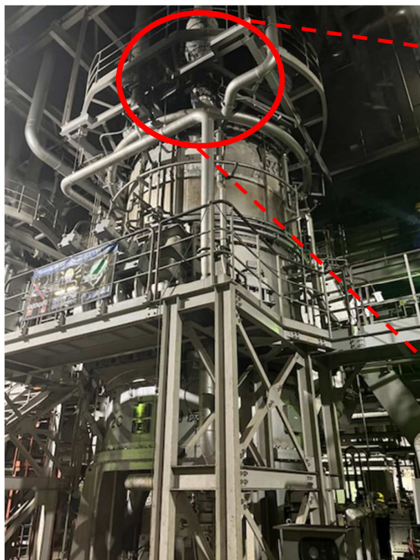
火災が発生した微粉炭機 (全景)
