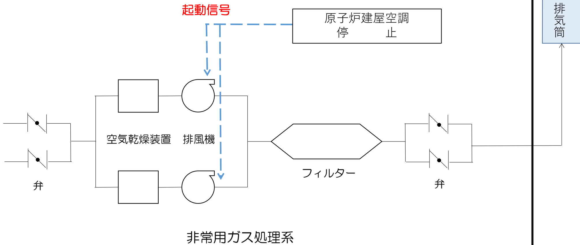
図 非常用ガス処理系の計画外作動の状況（イメージ図）
