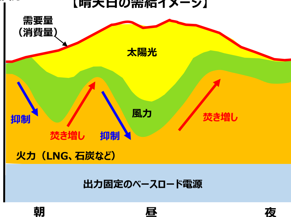
発電出力
