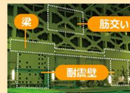
オベーションフロアの天井(左)・壁面(右)の耐震補強
