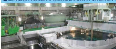
②燃料装荷(写真は原子炉に燃料集合体を挿入する作業の様子)
