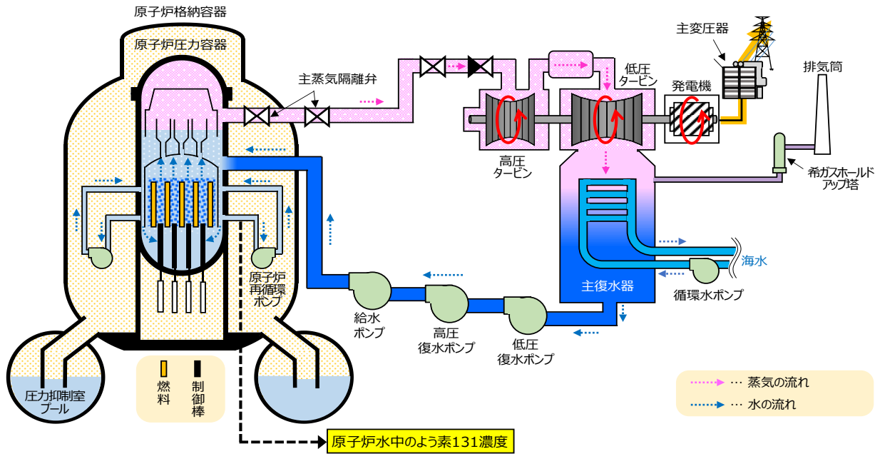
女川原子力発電所2号機 概略図
