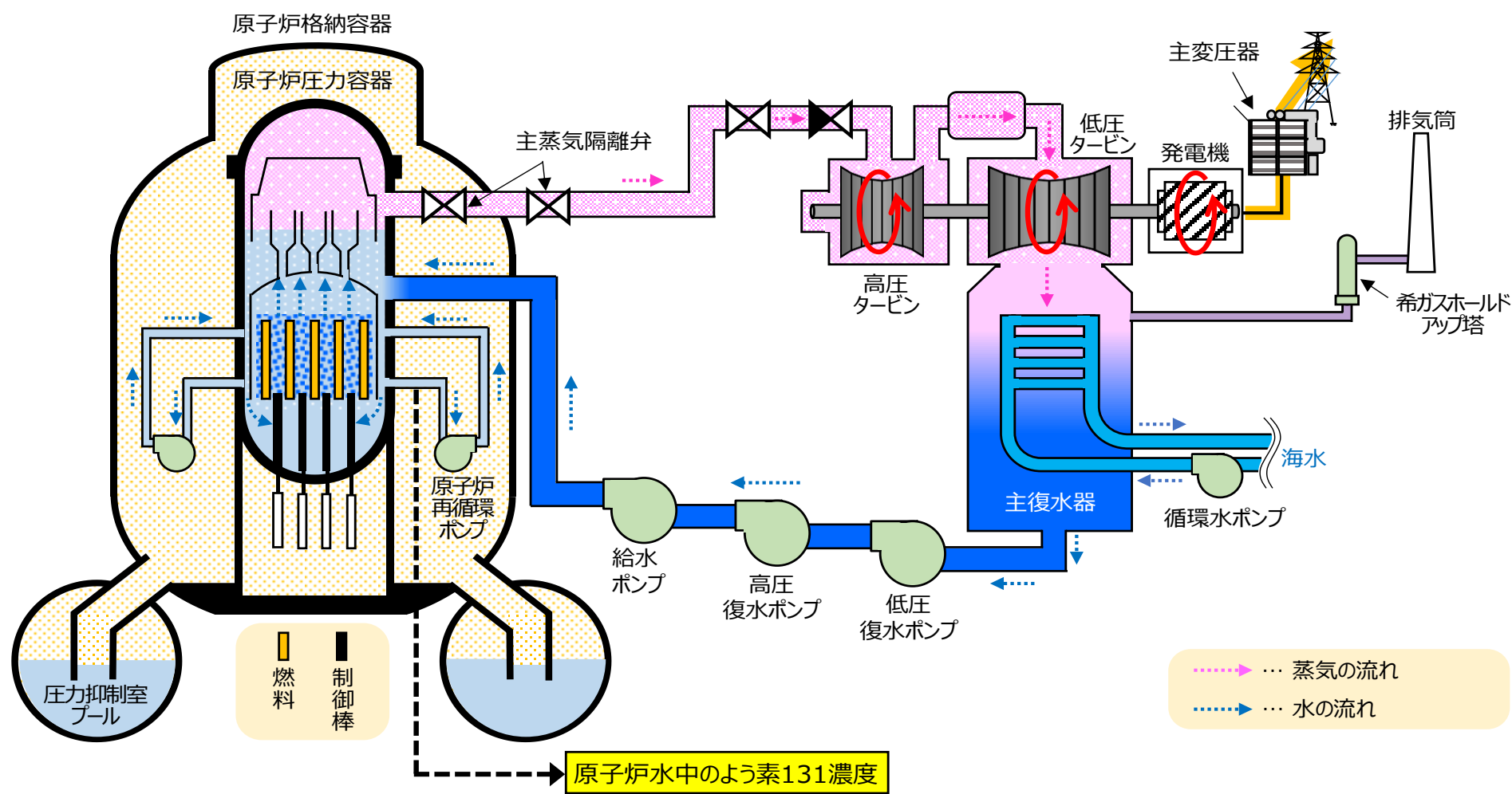
女川原子力発電所 2号機 概略図
