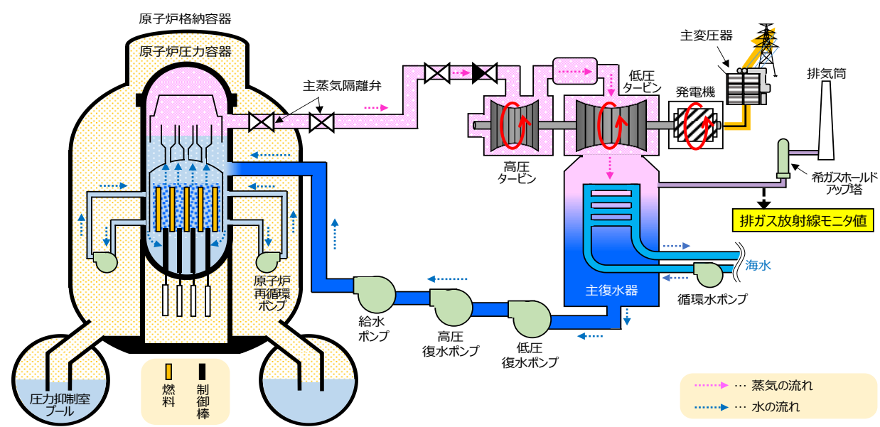
女川原子力発電所 2号機 概略図
