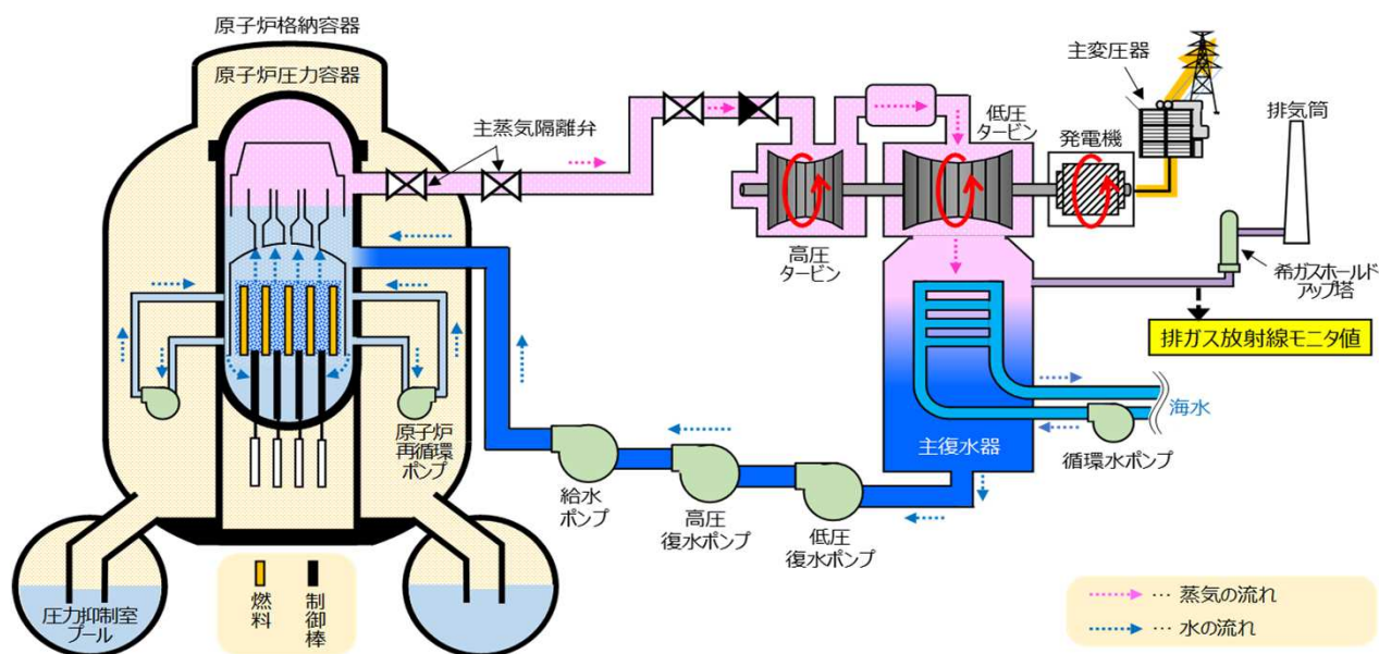
女川原子力発電所 2号機 概略図
