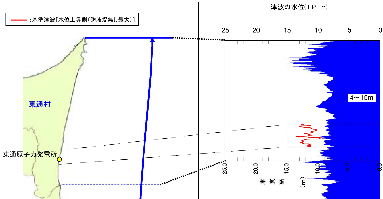
基準津波[水位上昇側(防波堤無し最大)]と青森県海岸津波対策検討会(2012)による東通発電所周辺の海岸線上の津波水位の比較※ (青森県海岸津波対策検討会(2012)に一部加筆)
