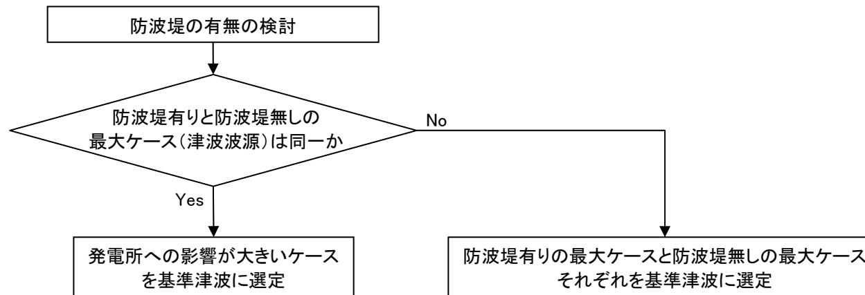
[基準津波の選定フロー]
