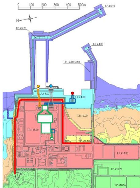
津波水位の評価位置
