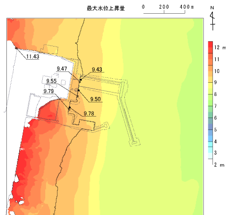
基準津波 [水位上昇側(防波堤無し最大)]
