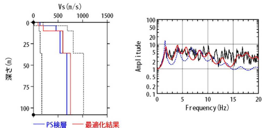
伝達関数の比較(水平)
