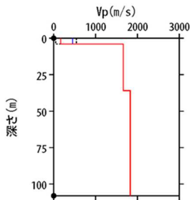
— PS検層 — 最適化結果
