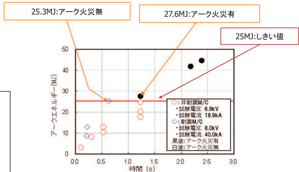
参考図3-1 試験結果(アーク火災発生状況)
