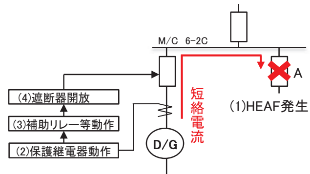
A: M/C 6-2Cに接続される遮断器 (非常用ディーゼル発電機(A)受電遮断器52-6-2DGAを除く。)
