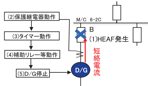
B: 非常用ディーゼル発電機(A)受電遮断器52-6-2DGA
