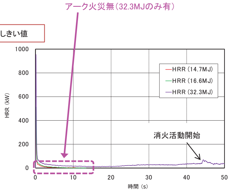
参考図3-7 発熱速度(HRR)測定結果 (M/C(D/G)試験時)
