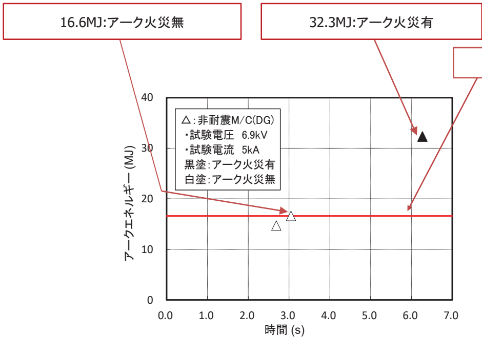
参考図3-6 試験結果(アーク火災発生状況)
