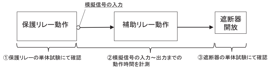
参考図8-1 M/Cに接続される遮断器（D/G受電遮断器以外）でのHEAF時
