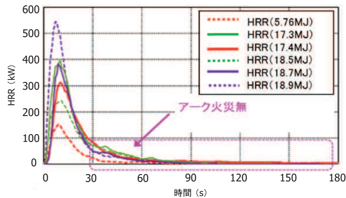
参考図3-3 発熱速度(HRR)測定結果 (P/C試験時)
