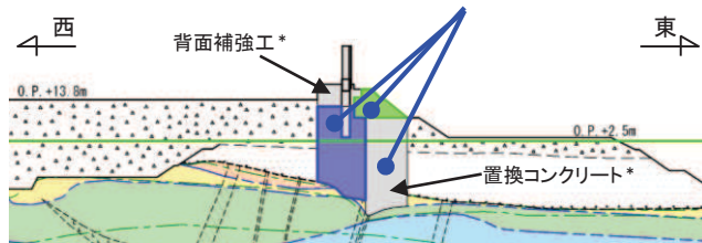
防潮堤(鋼管式鉛直壁一般部)
