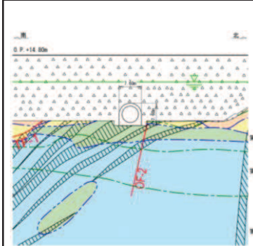
断面①
