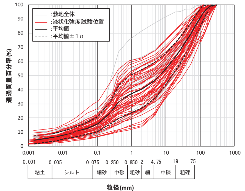
粒度分布の確認結果
