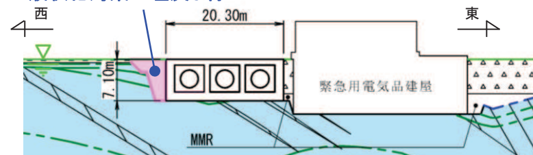
ガスタービン発電設備軽油タンク室(東西)
