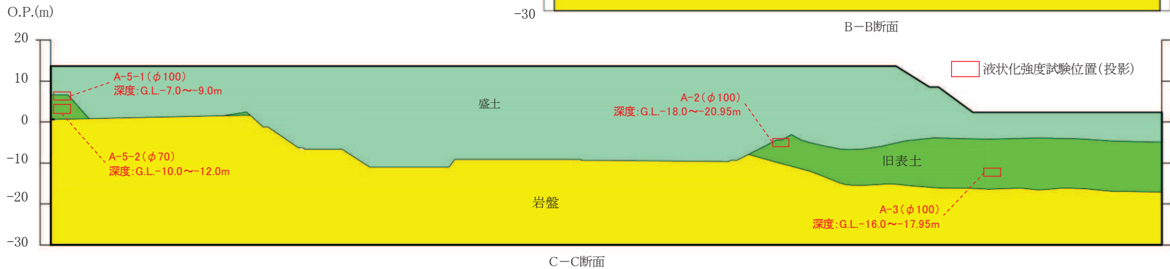
旧表土の液状化強度試験の試料採取位置(1/2)
