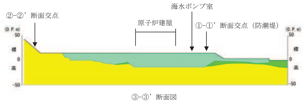
盛土及び旧表土の分布断面図
