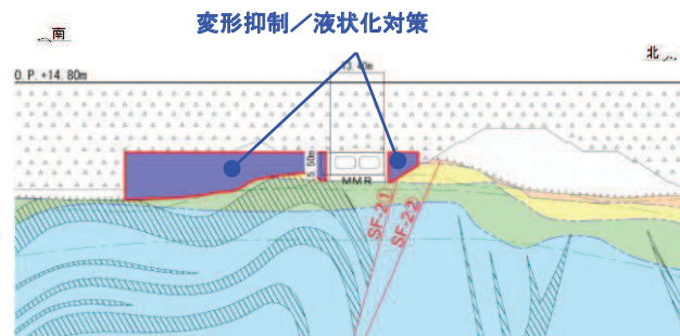
取水路(標準部)(断面⑥)
