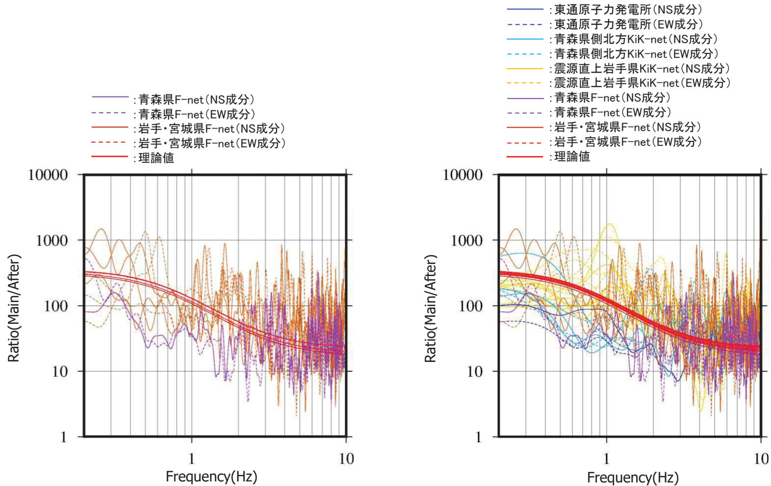
(1) F-net観測点
