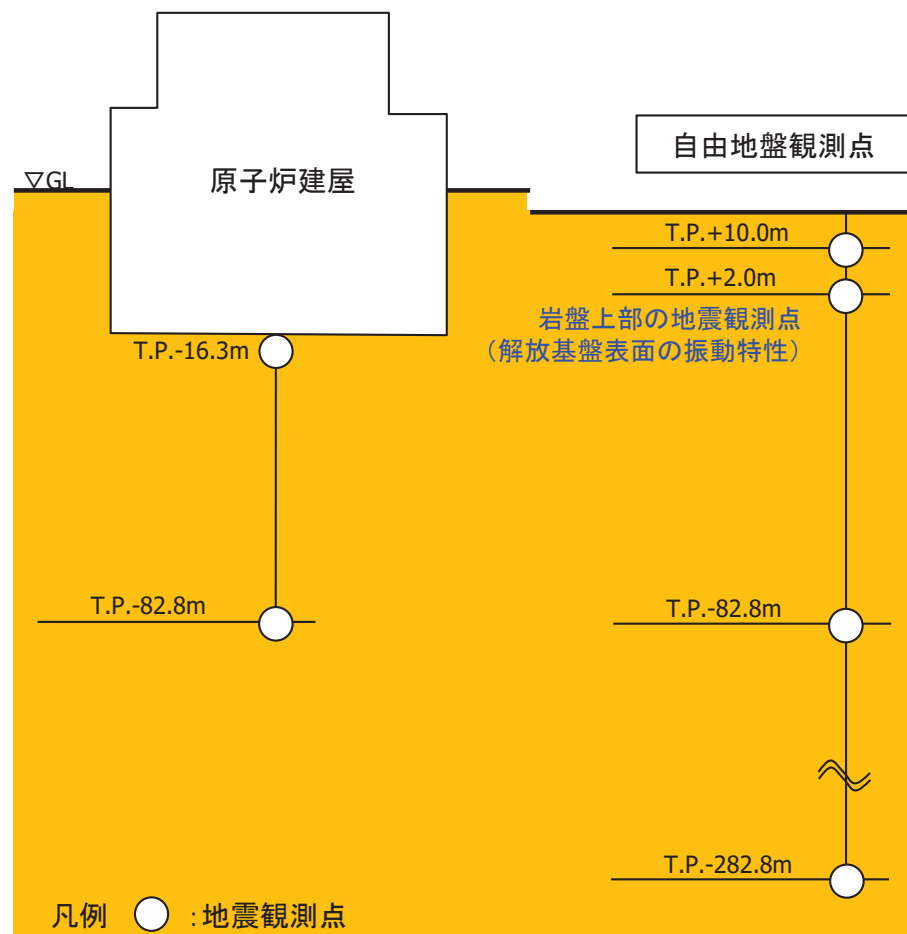
敷地内地盤系の地震観測点
