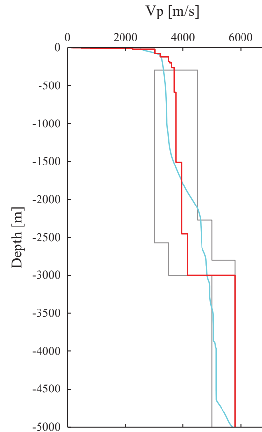
推定された鉛直分布 Vp
