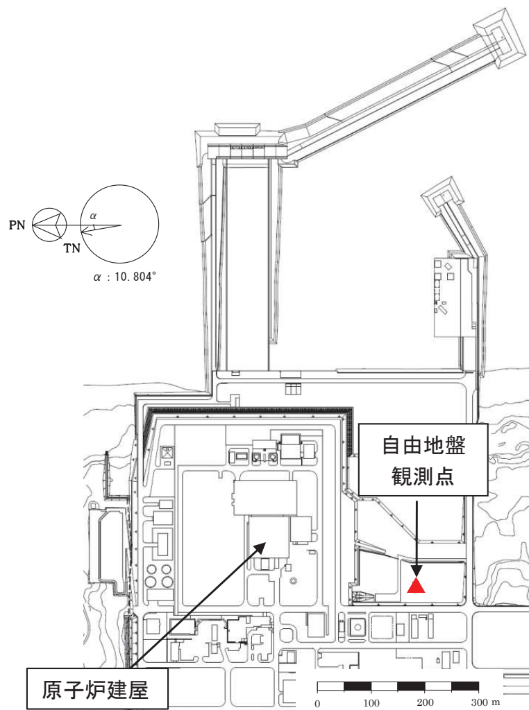
平面配置図
