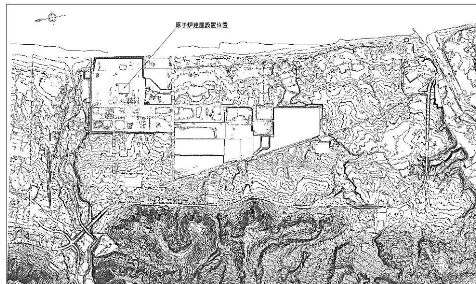
敷地のDEM地形図(敷地造成後)
