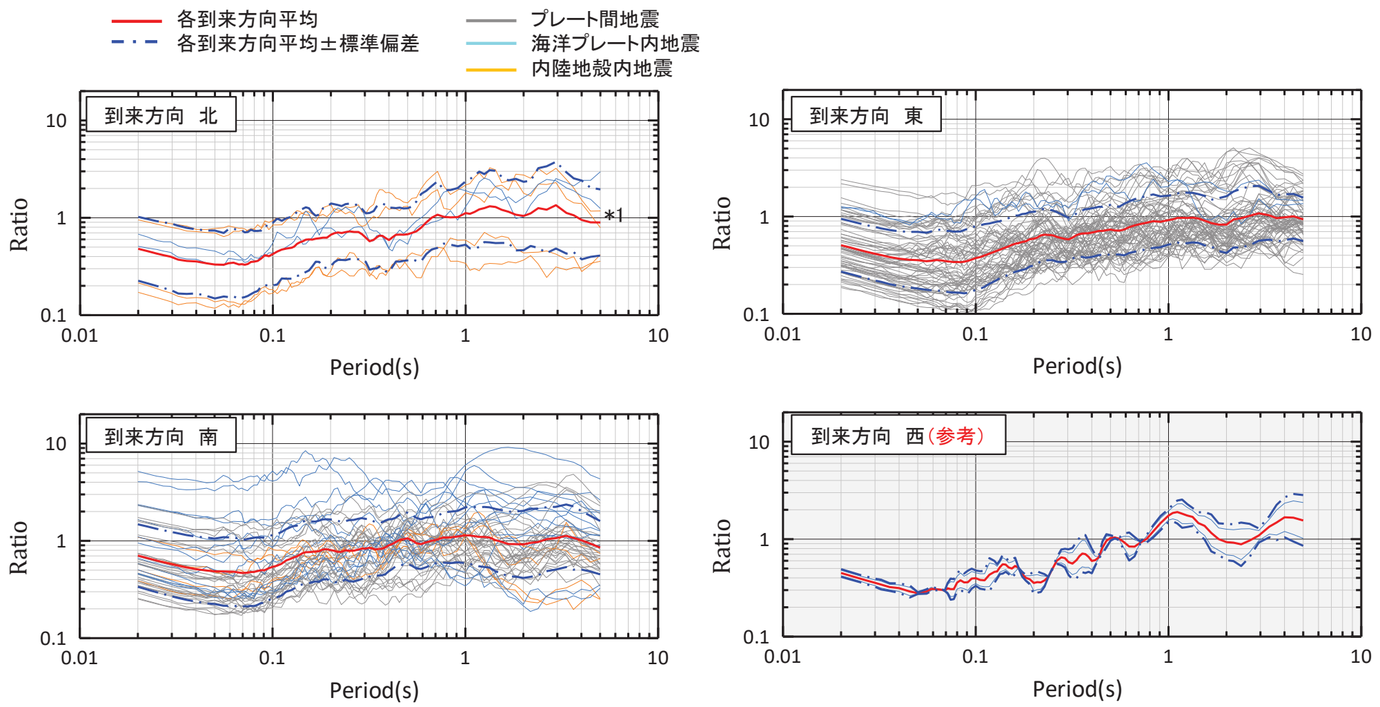
観測記録とNoda et al.(2002)との比較 地震波到来方向別 水平成分 自由地盤の岩盤上部地震観測点 (T.P.+2.0m) / Noda et al.(2002)
