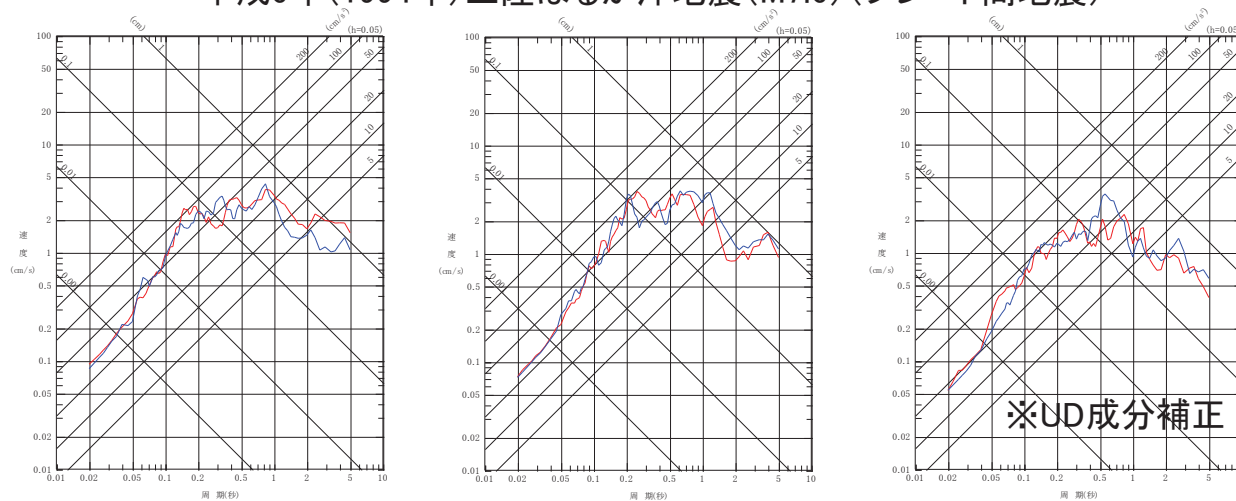
NS成分 EW成分 UD成分 2008年岩手県沿岸北部の地震(M6.8) (海洋プレート内地震)
