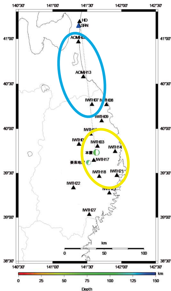
観測点位置図
