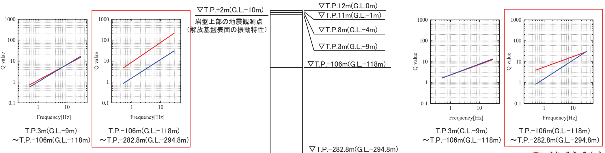
《推定された Q_s 》
