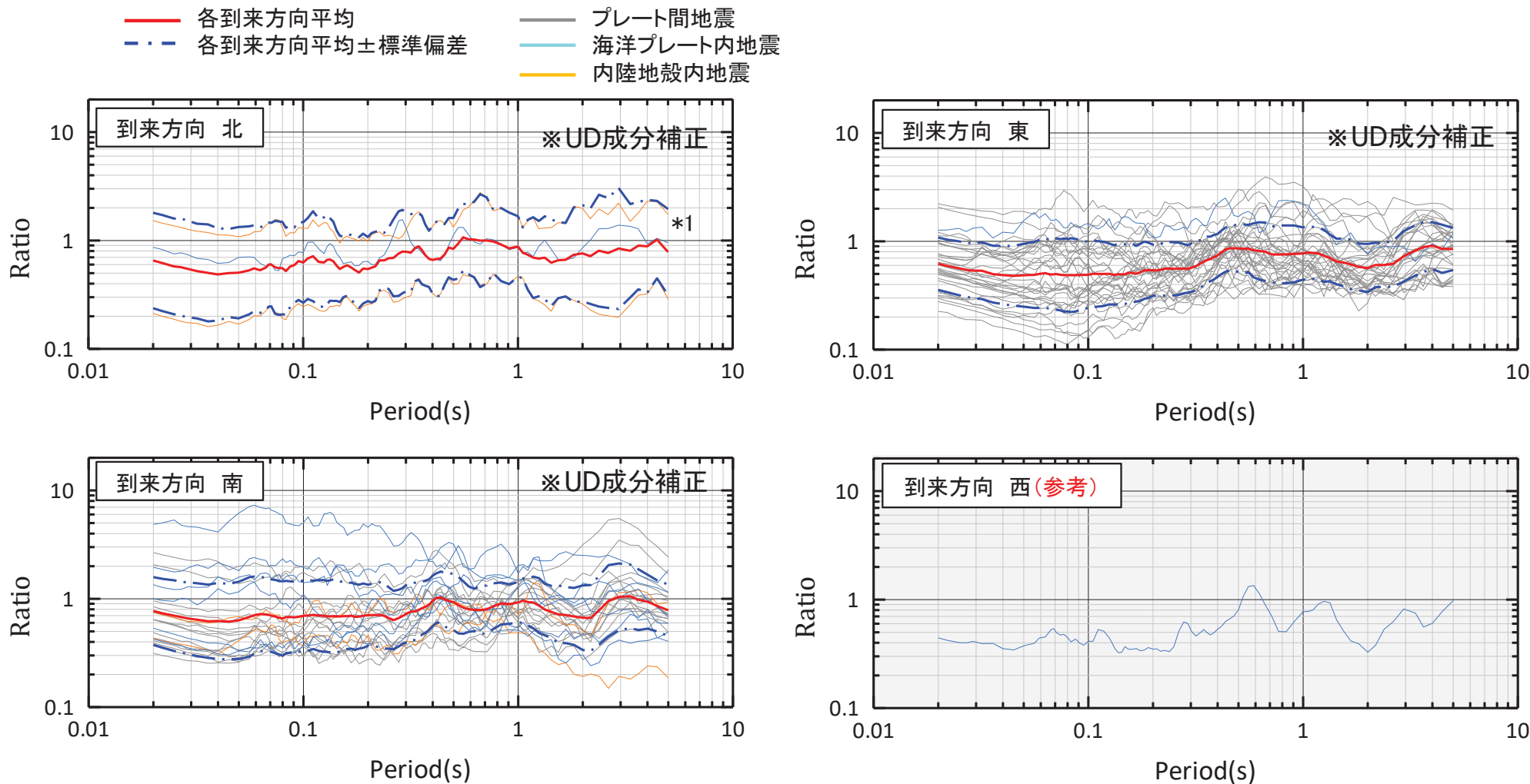
観測記録とNoda et al.(2002)との比較 地震波到来方向別 鉛直成分
