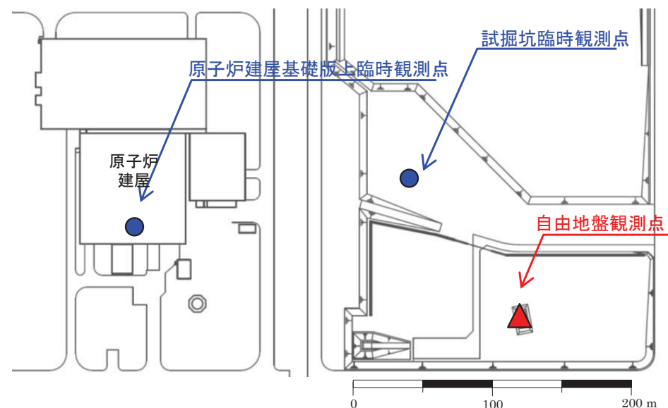
検討に用いた地震観測点
