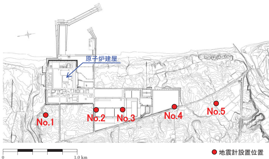
南北アレイ臨時観測の位置
