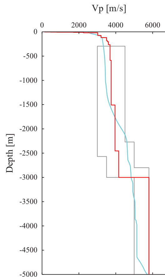
推定された鉛直分布 Vp
