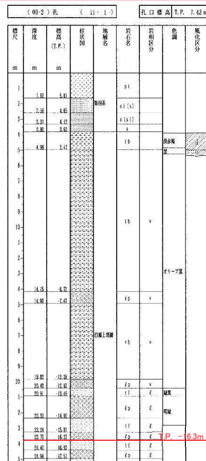
地質柱状図及びコア写真
