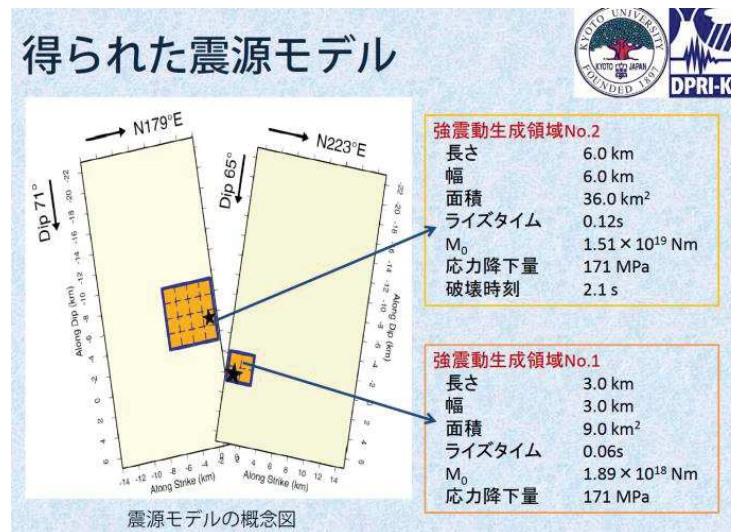
震源モデル
