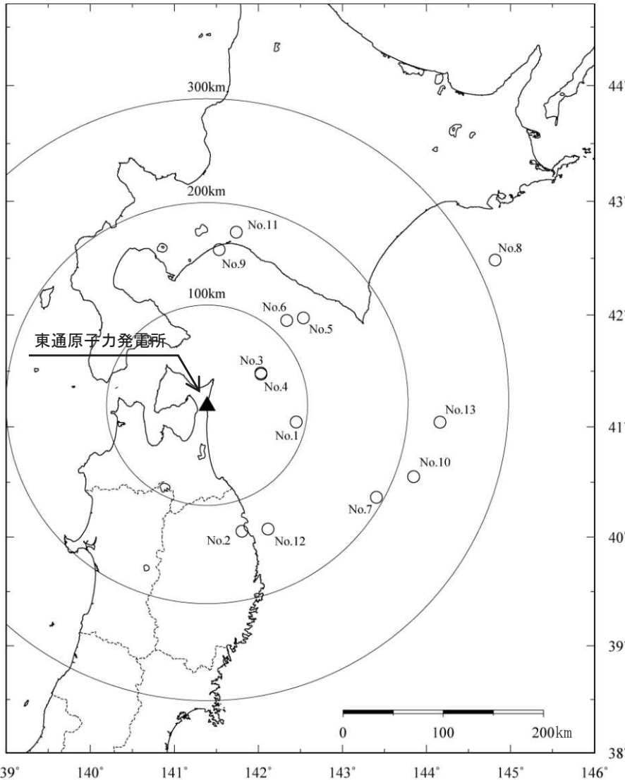
検討に用いた観測地震の震央分布
