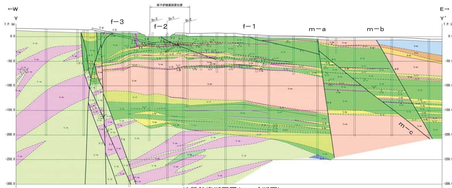
地質鉛直断面図(Y-Y'断面)
