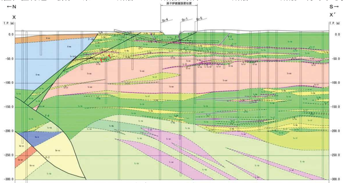
地質鉛直断面図(X-X'断面)
