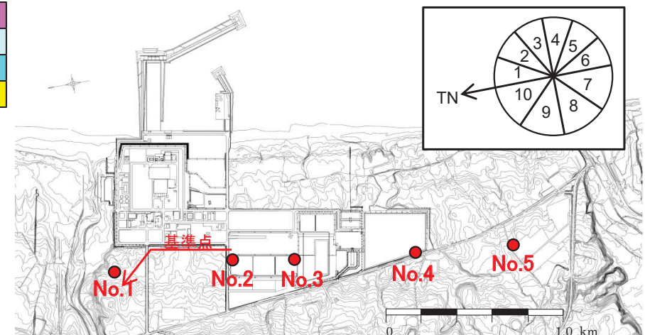
キープランと地震の方位区分
