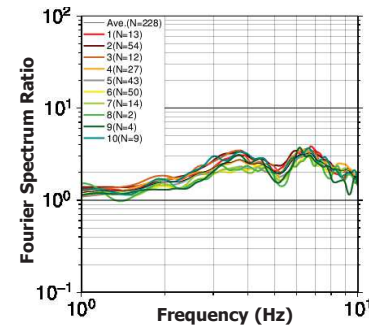
基準化スペクトル(例) (地震波到来方向の比較)
