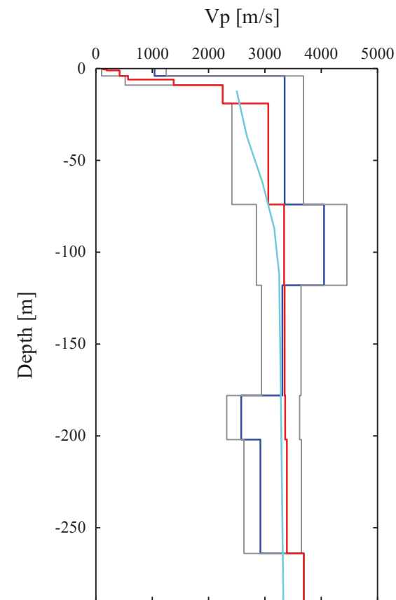
《 推定された鉛直分布 Vp 》
