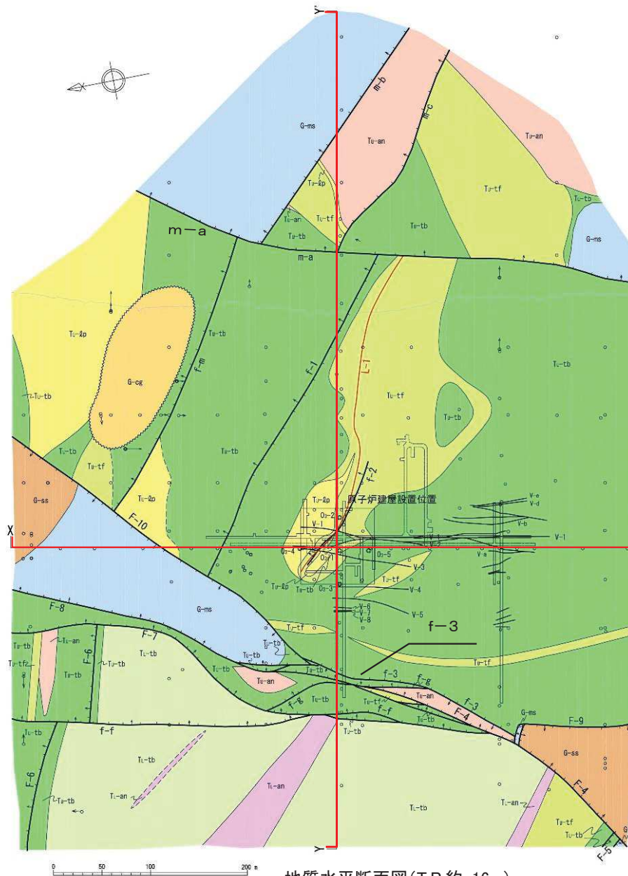
地質水平断面図 (T.P.約-16m)
