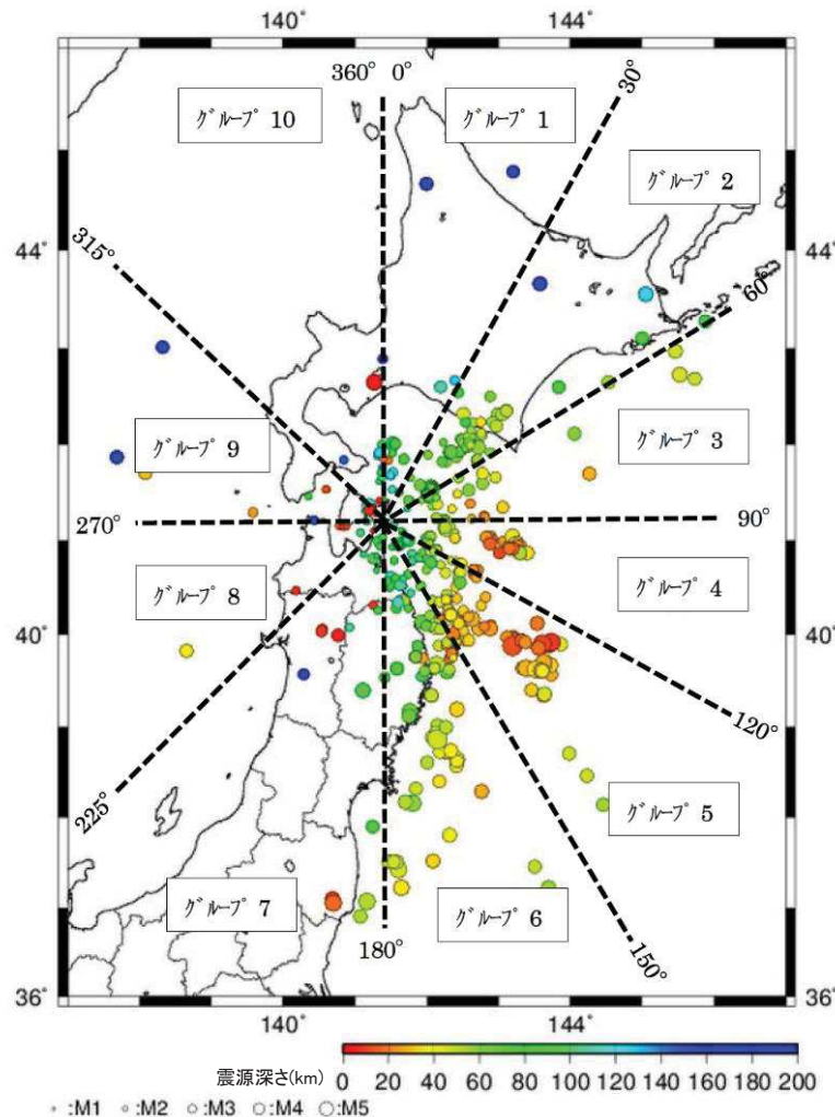
観測地震の震央分布と方位区分
