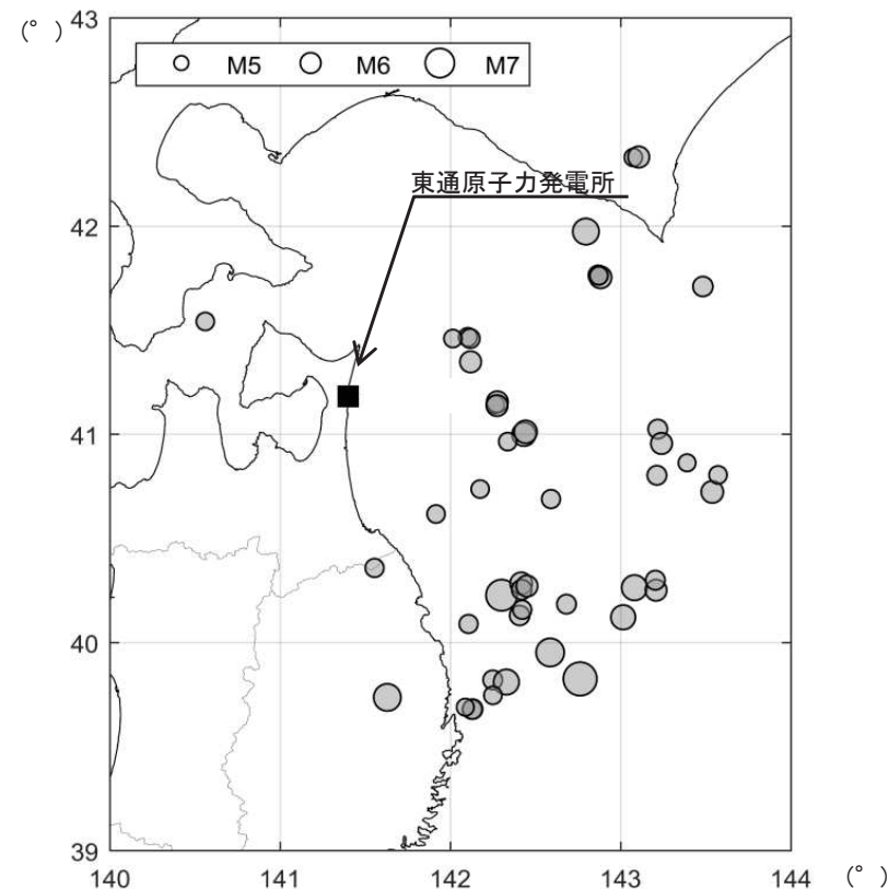
震央分布
