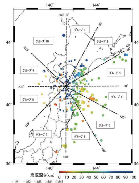
観測地震の震央分布と方位区分
