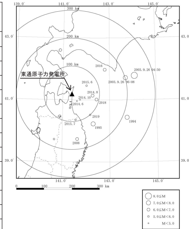
震央分布図
