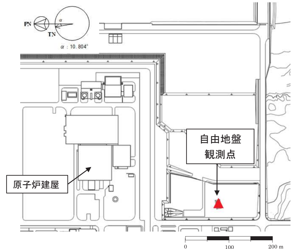
検討に用いた地震観測点
