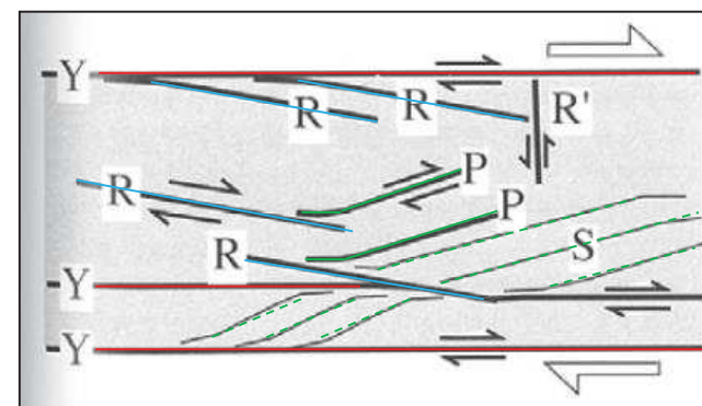
脆性断層岩に見られるせん断組織(右横ずれの場合)
