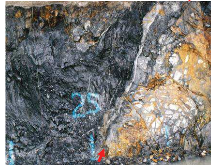
直掘部法尻のTF-6断層 N57° W80° SW(上盤)~N63° W/87° SW (下盤)。黒色の葉片状部(幅1cm以下)を伴う。
