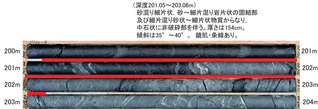
1Rsy-4孔(斜め60° ボーリング)コア写真
