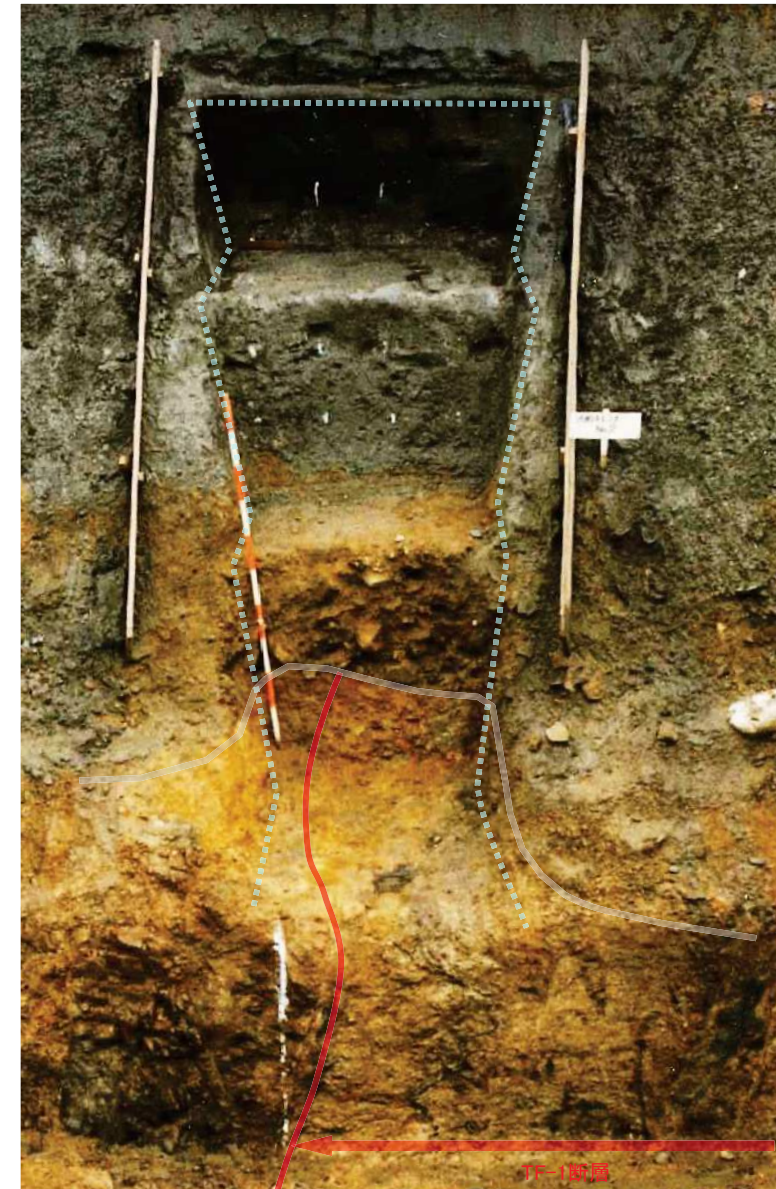
TF-1断層調査トレンチ露頭(露頭写真)
