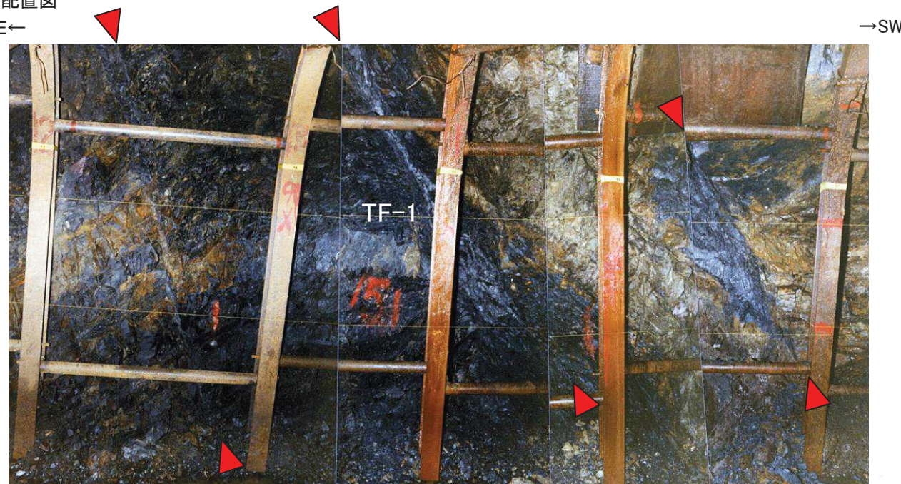
TF-1断層 2号炉試掘坑B坑南東壁写真
