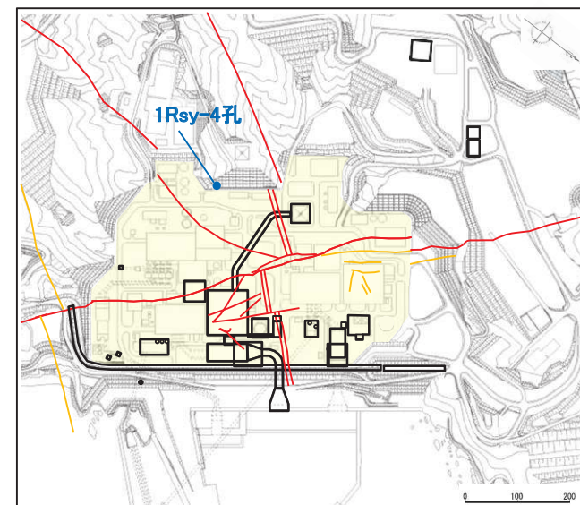
ボーリング位置図(1Rsy-4孔)
