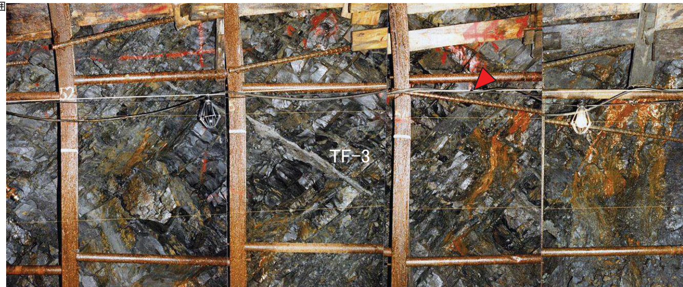
TF-3断層 2号炉試掘坑B坑北西壁写真
