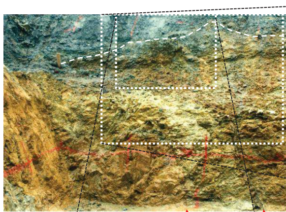
TF-1断層破碎帯下盤側境界と 第四系基底面との関係 (南側法面: 追い込み掘削前)
