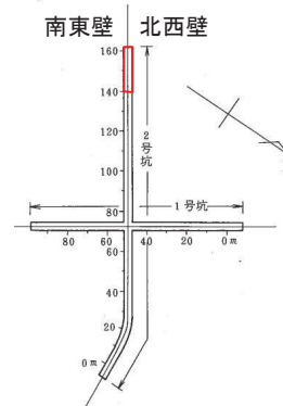
試掘坑配置図
