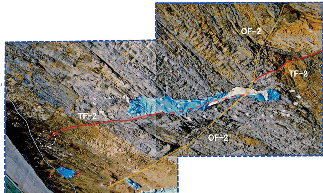
2号原子炉建屋掘削時の岩盤状況写真 (写真は天地を反転)
