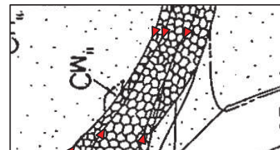
TF-1断層近傍 3号炉試掘坑2号坑北西壁スケッチ (展開図を反転)
