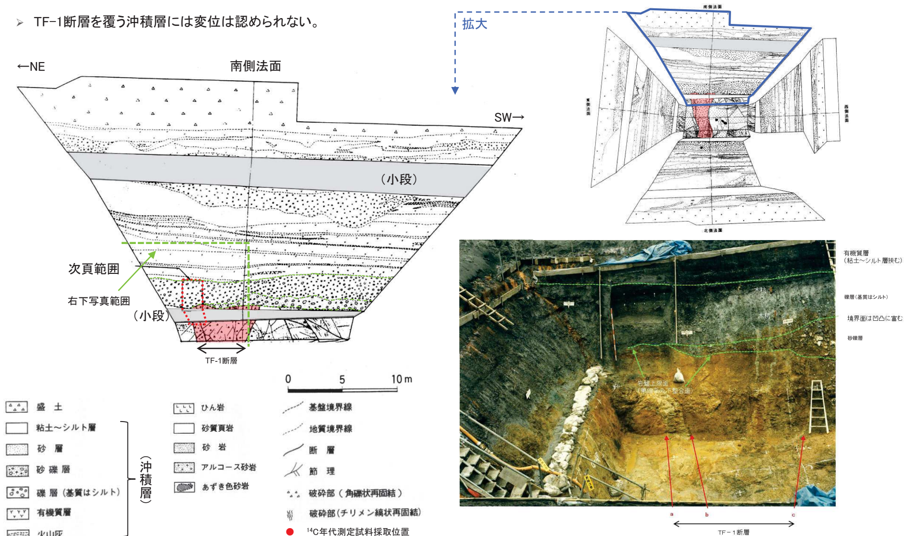
TF-1断層調査トレンチ露頭スケッチ(南側)
