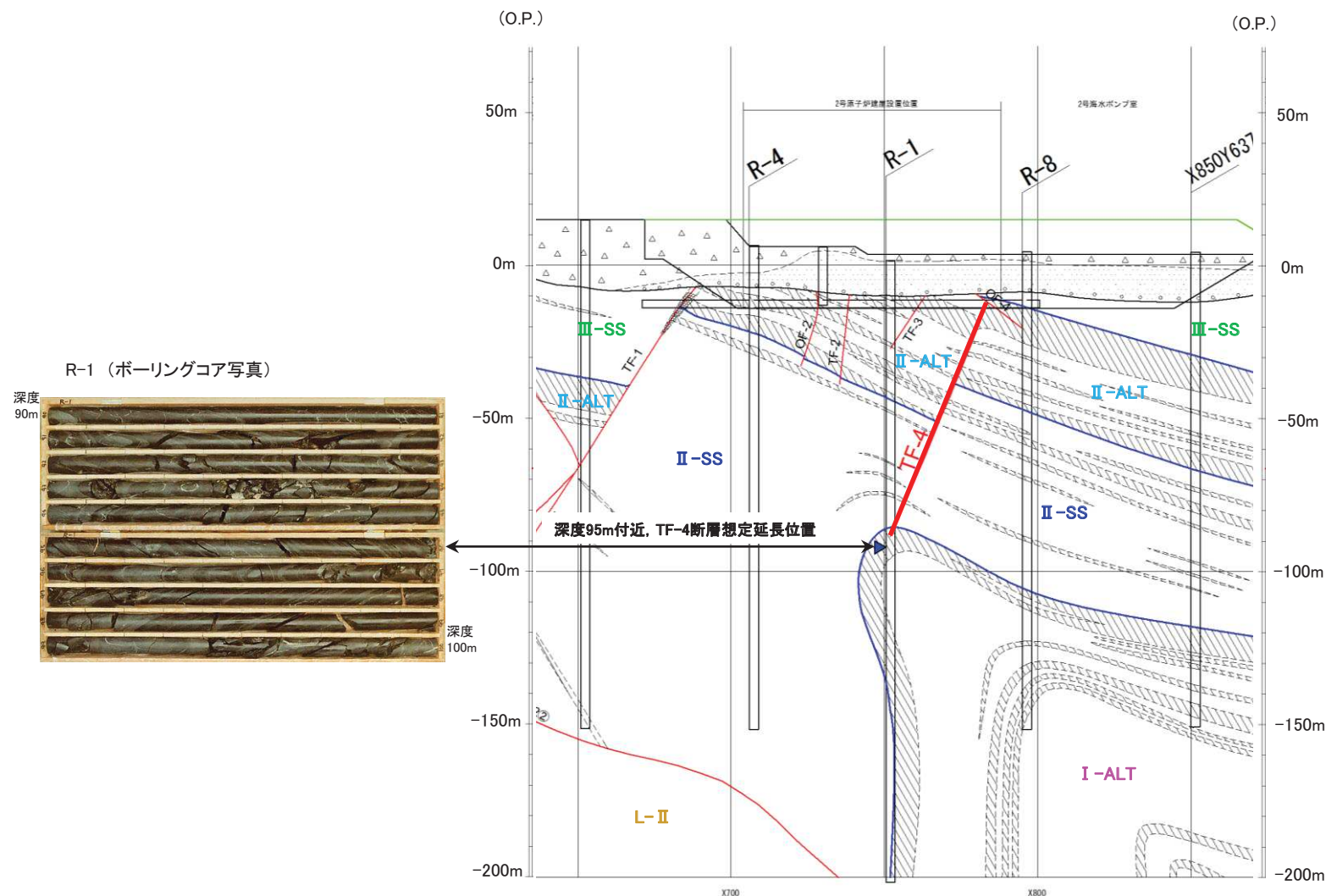
TF-4断層の連続性検討図 (2号炉心Y-Y'断面)
