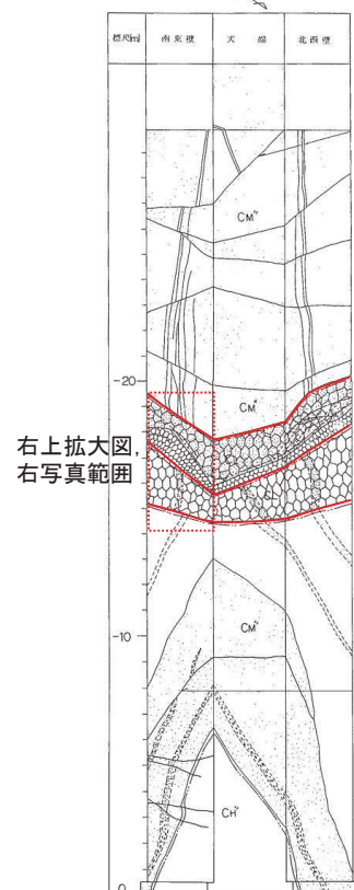
TF-1断層周辺 2号炉試掘坑B坑展開図
