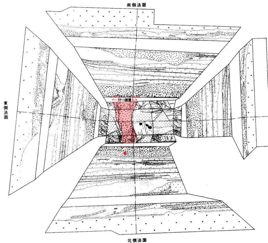
TF-1断層調査トレンチ露頭スケッチ(全体)
