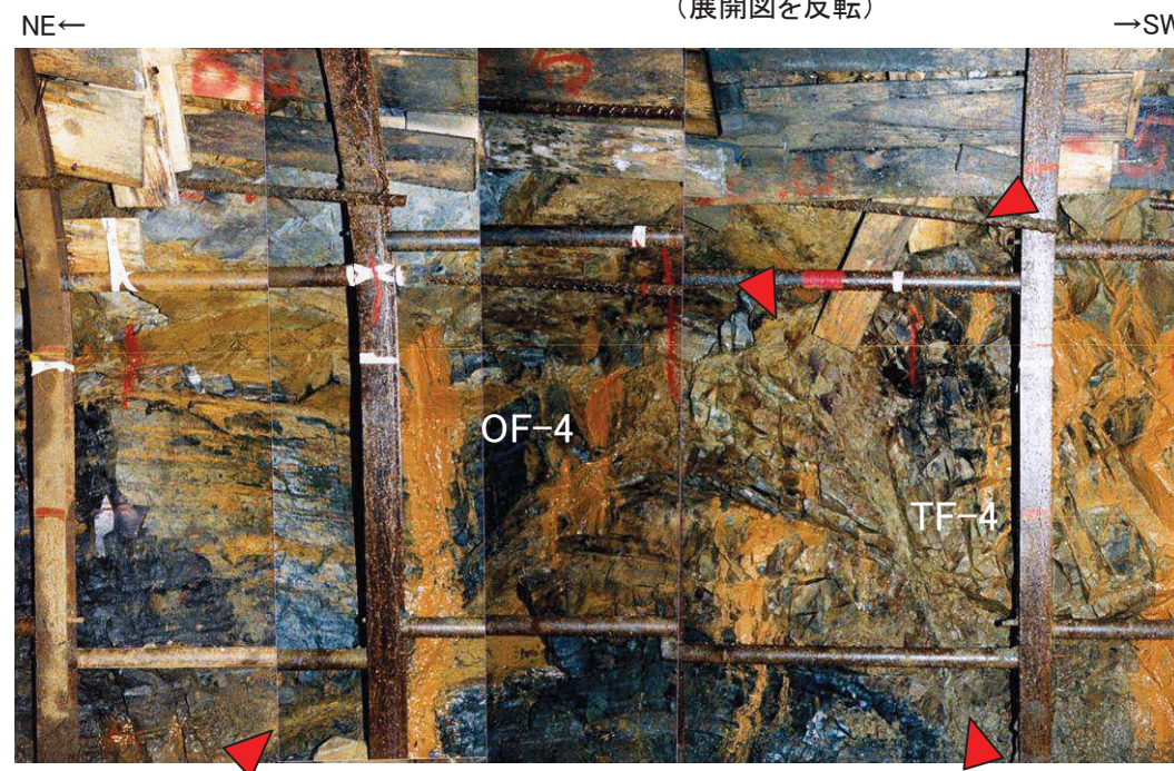
OF-4断層、TF-4断層 2号炉試掘坑B坑南東壁写真
