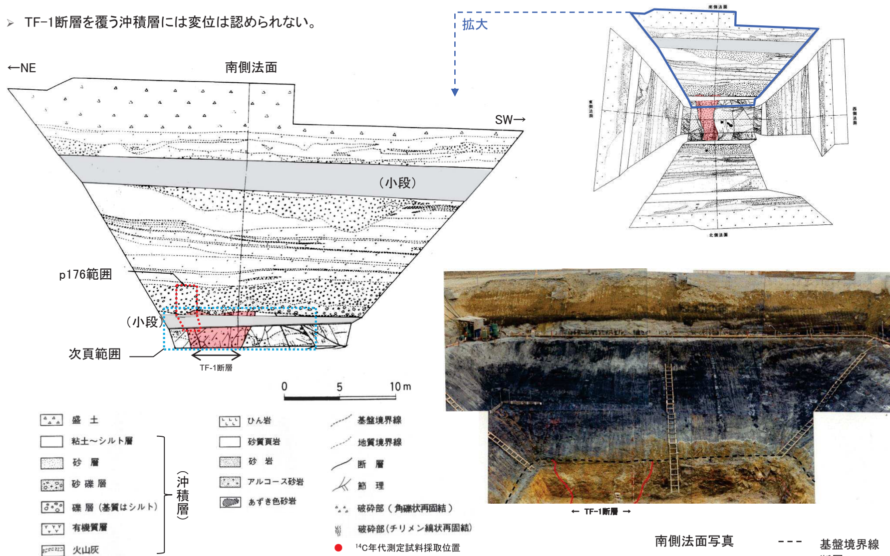
TF-1断層調査トレンチ露頭スケッチ(南側)
