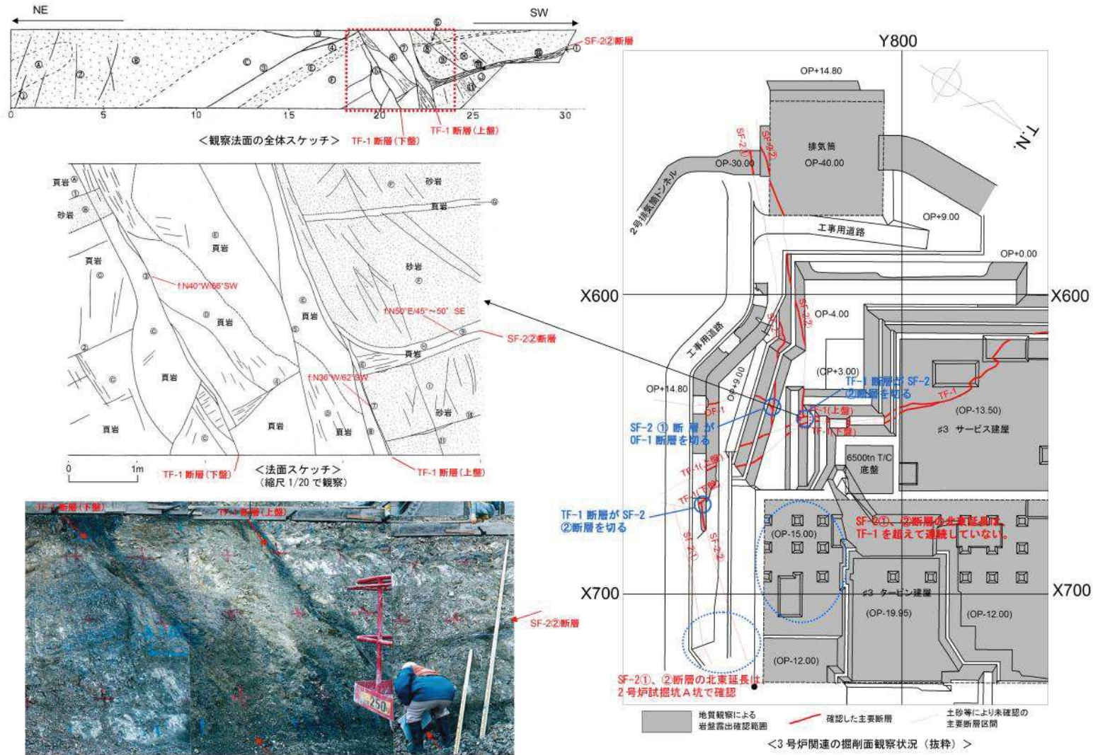
<TF-1断層(上盤)がSF-2断層を切る状況>
