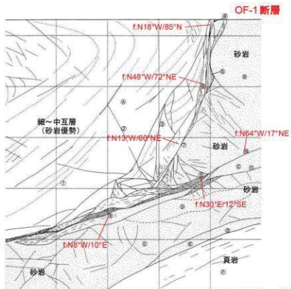
<SF-2①断層とOF-1断層の会合状況>
