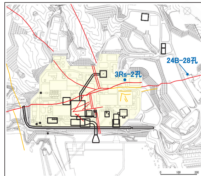
ボーリング位置図(3Rs-2孔, 24B-28孔)
