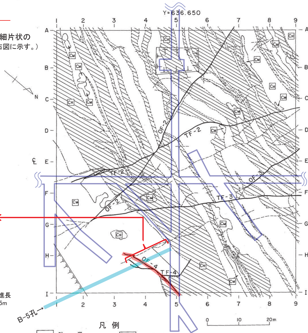
2号原子炉建屋掘削底盤スケッチ
