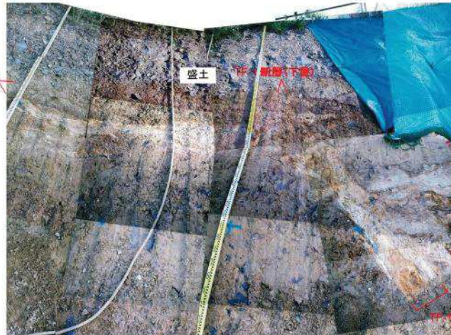
<TF-1断層(下盤)がSF-2断層を切る状況>
