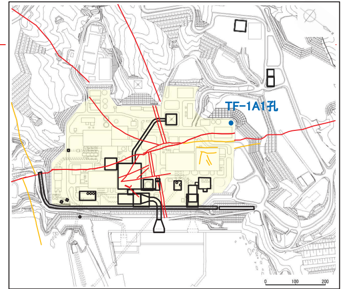
ボーリング位置図 (TF-1A1孔)
