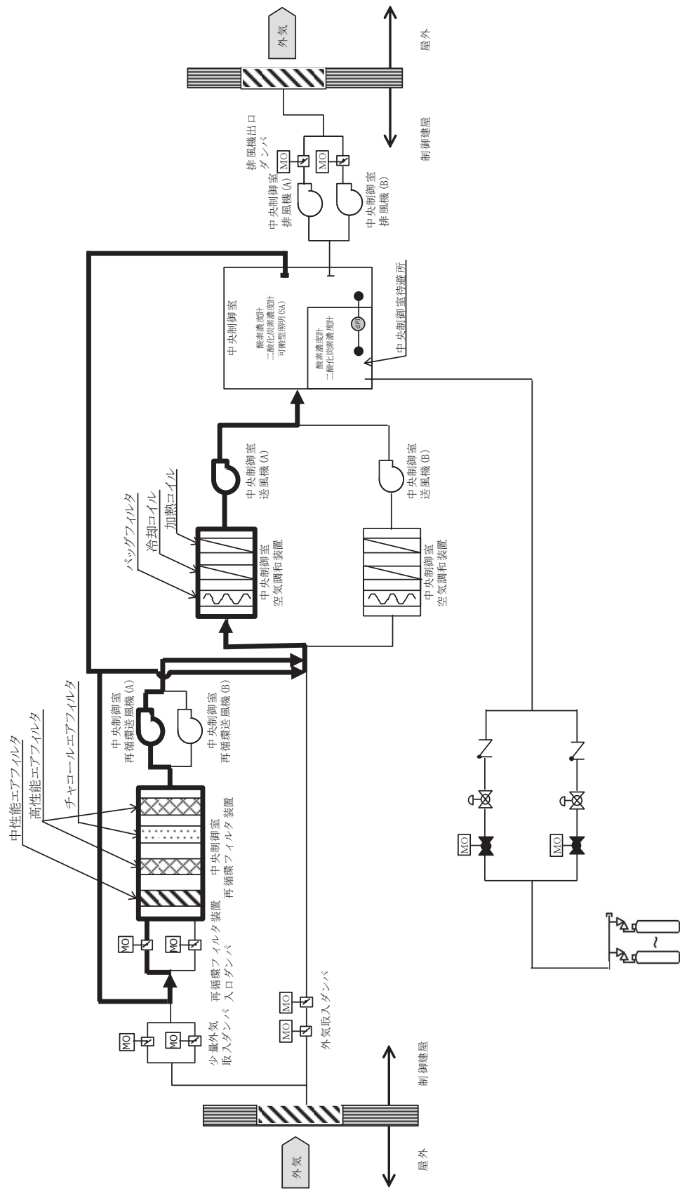
中央制御室待機所加圧設備 (空気ポンプ)
